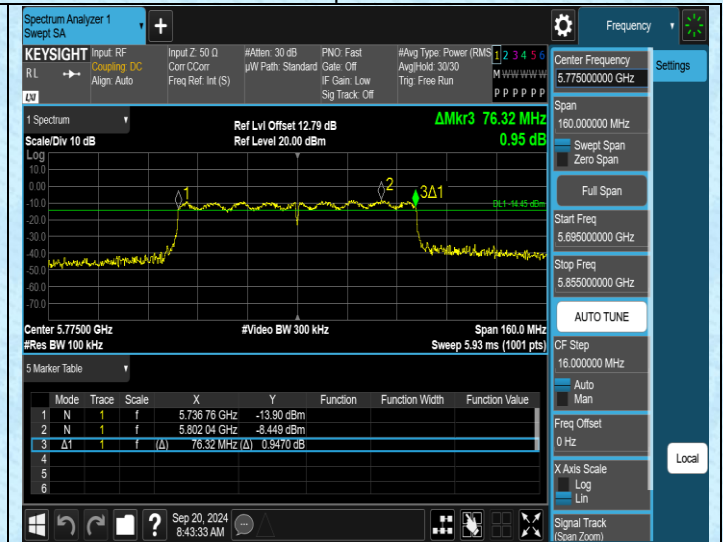
11AC80SISO-Ant1-5775-PASS
