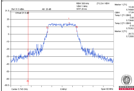
802.11a_Chain2 / CH149
