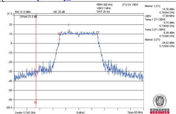
802.11ac(VHT20)_Chain3 / CH149
