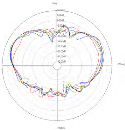
ZX-plane
