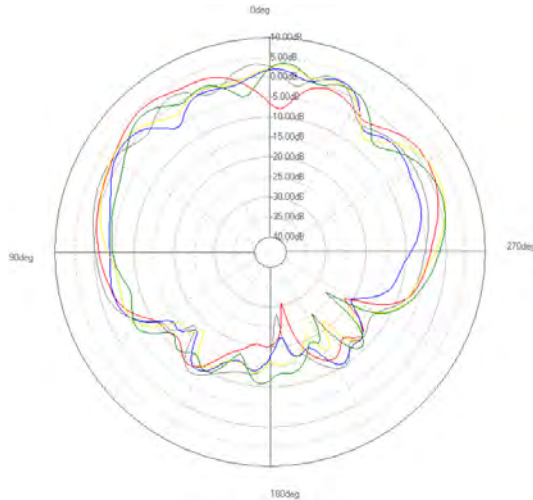
ZY-plane
