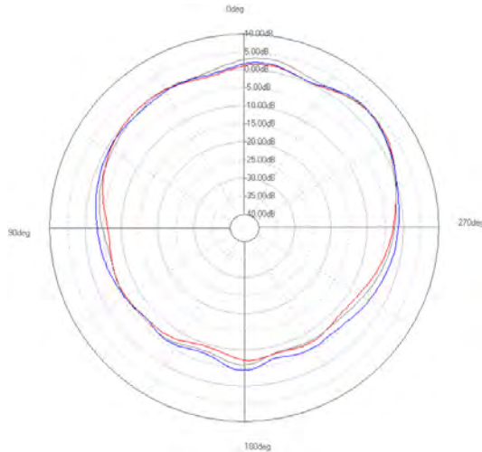
ZX-plane
