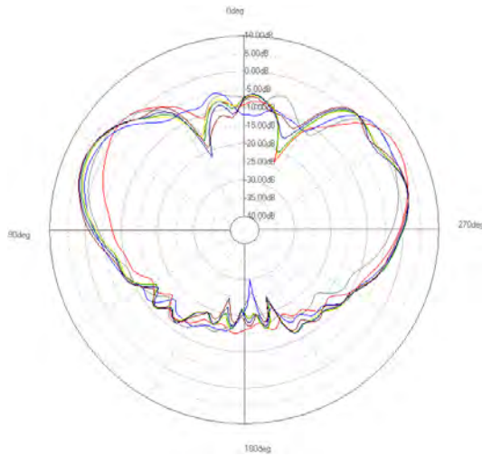
ZY-plane
