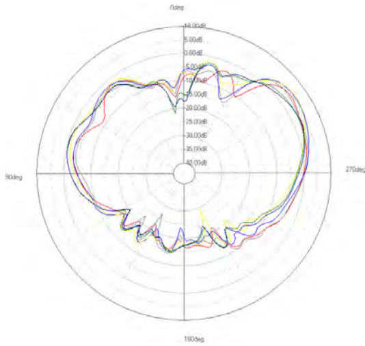
ZX-plane
