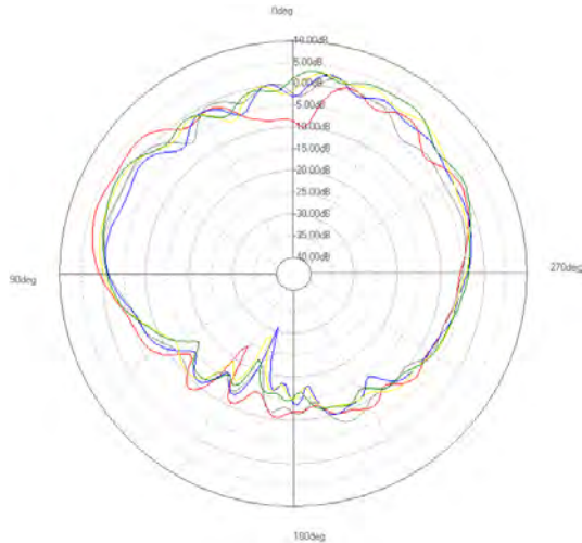
ZY-plane
