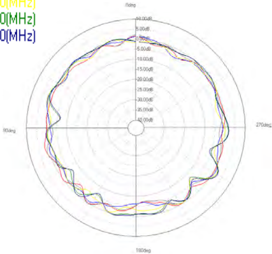
XY-plane
