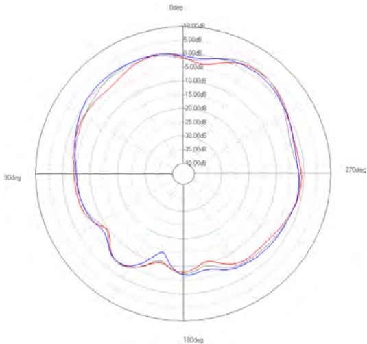
ZY-plane
