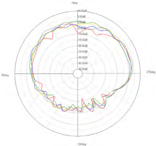
ZX-plane
