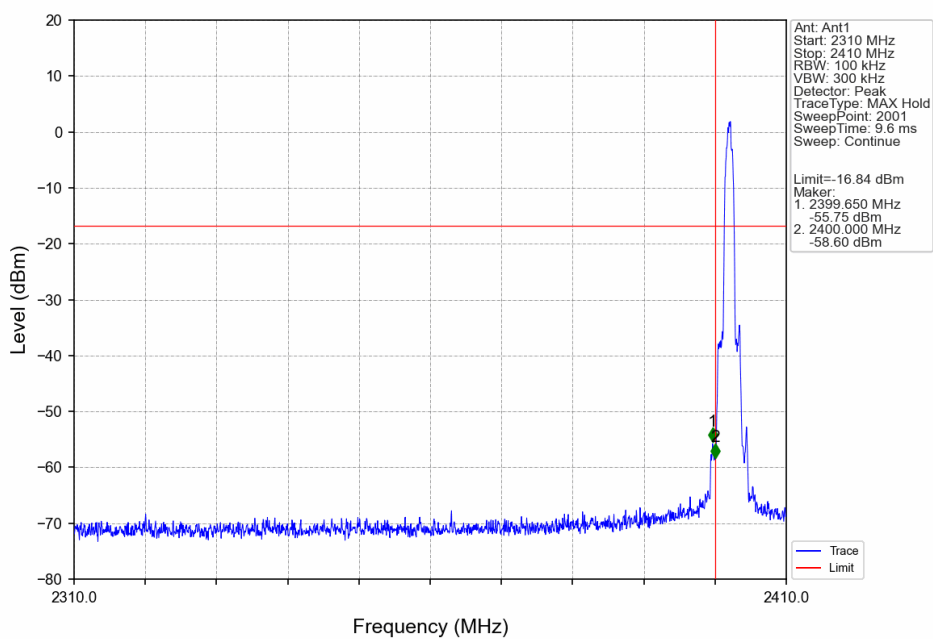
8DPSK 3DH5 LCH 2402MHz Ant1 NTN
