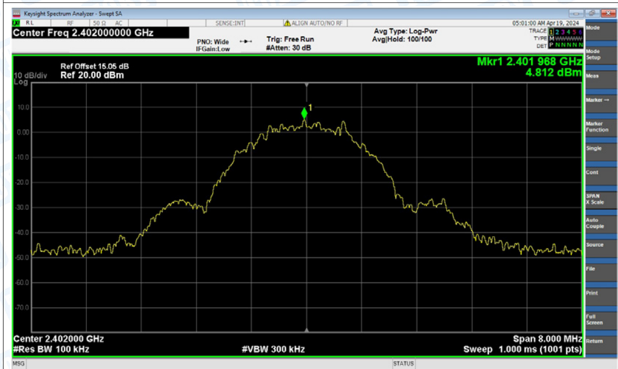
Band Edge NVNT BLE 2Mbps 2402MHz Ant1 Emission
