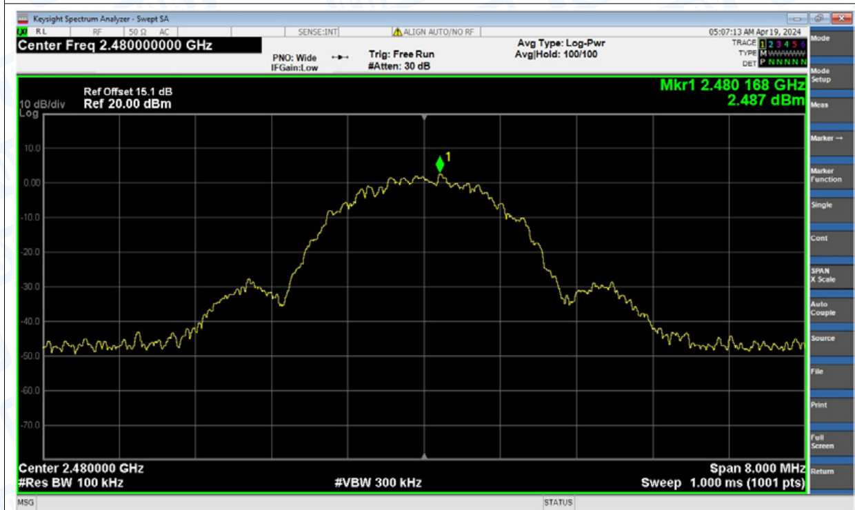
Band Edge NVNT BLE 2Mbps 2480MHz Ant1 Emission
