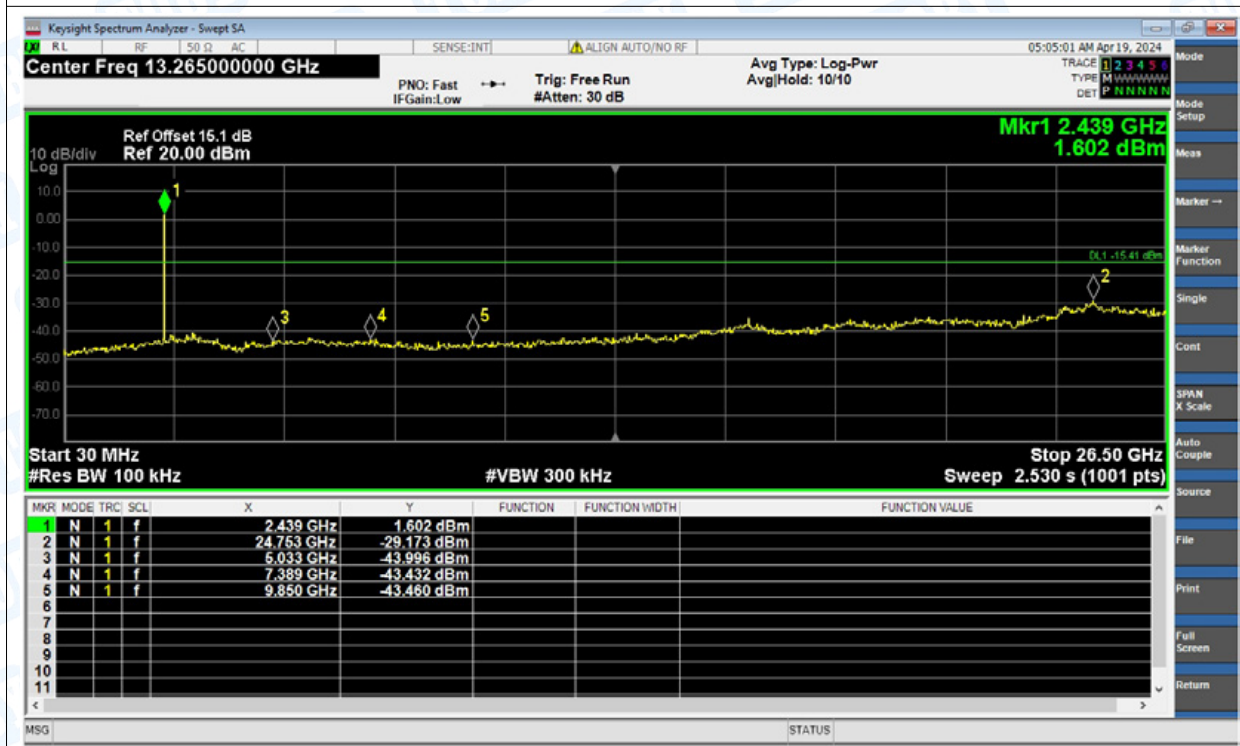
Tx. Spurious NVNT BLE 2Mbps 2440MHz Ant1 Emission
