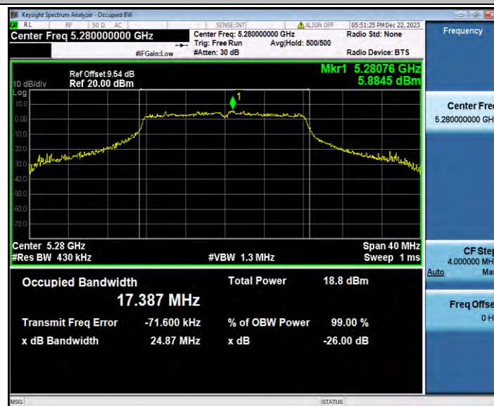
11A_Ant0_5280
