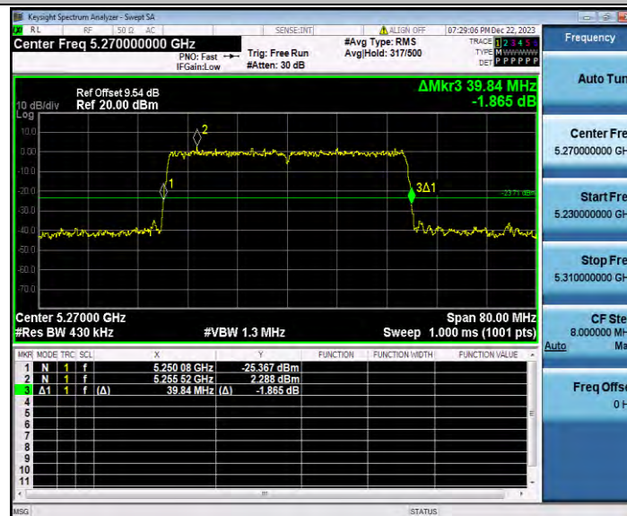
11AX40SISO_Ant0_5270
