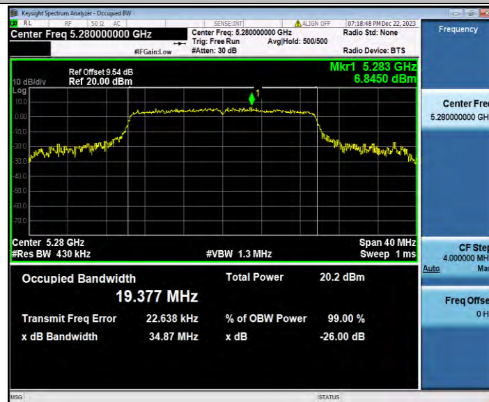
11AX20SISO_Ant0_5280
