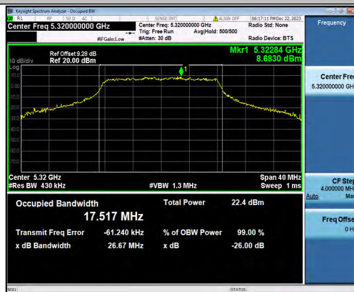
11N20SISO_Ant0_5320
