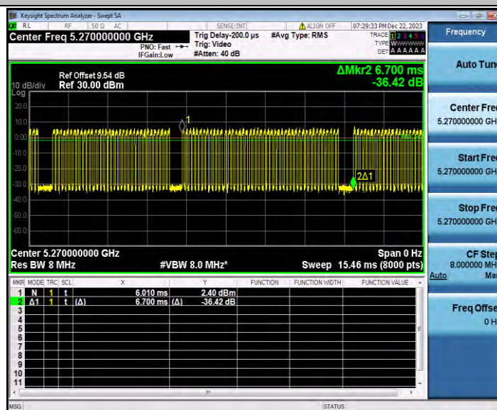
11AX40SISO_Ant0_5270
