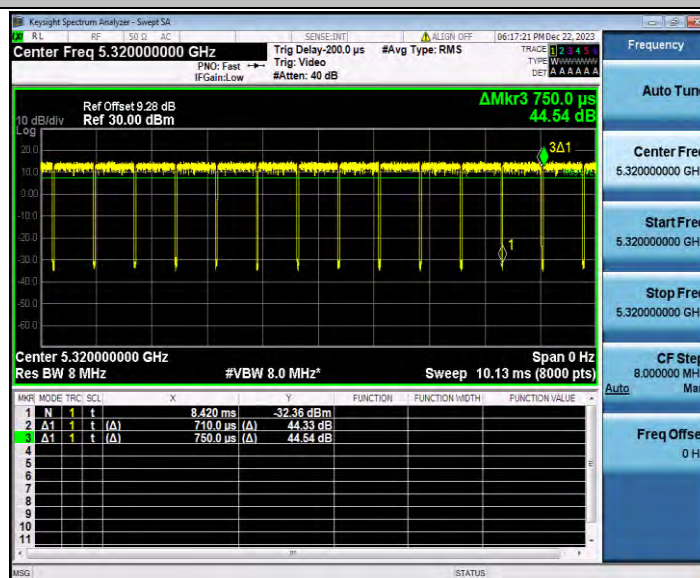
11N20SISO_Ant0_5320
