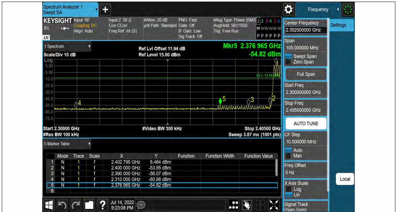
DH5_Ant1_Low_Hop_2402
