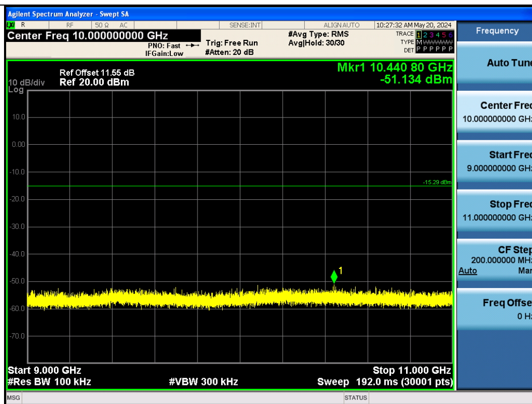
BLE_2M-Ant1-2440-9000~11000-PASS
