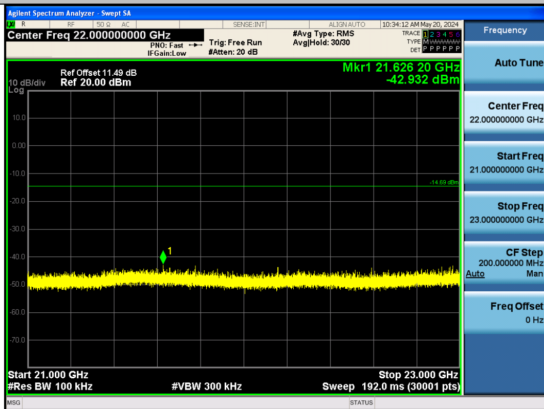
BLE_2M-Ant1-2480-21000~23000-PASS
