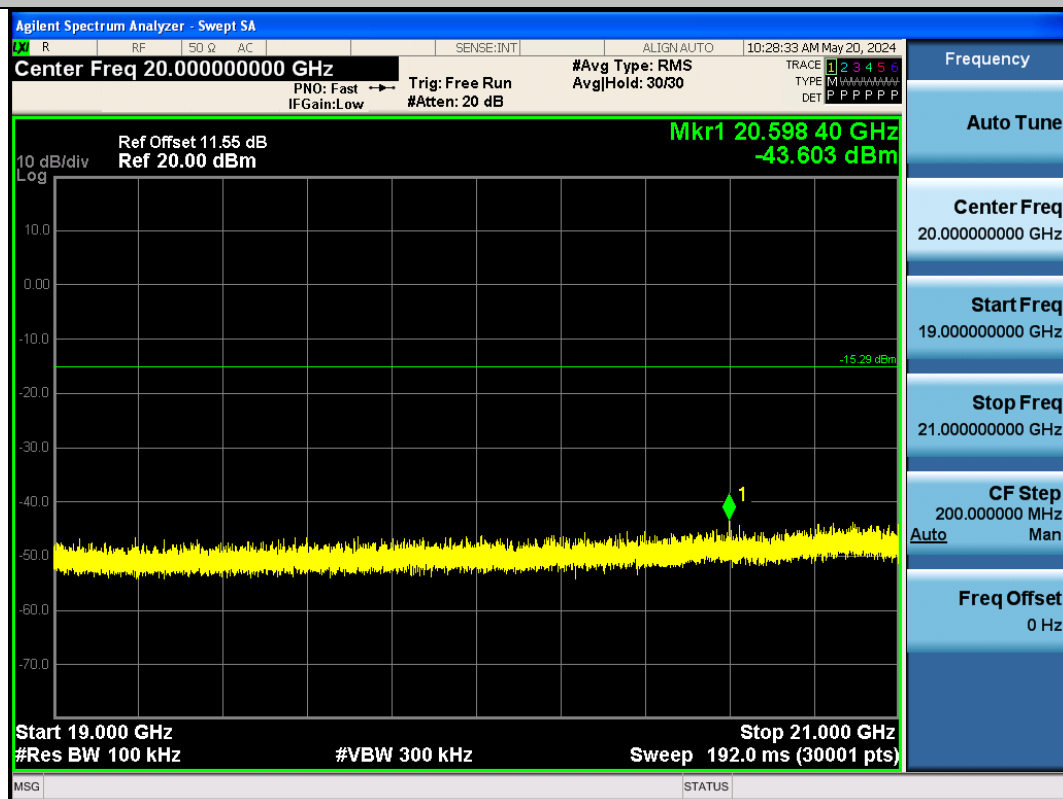
BLE_2M-Ant1-2440-19000~21000-PASS
