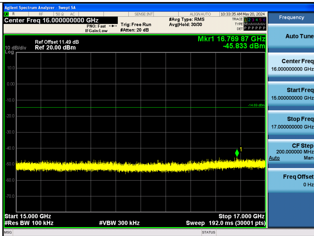
BLE_2M-Ant1-2480-15000~17000-PASS
