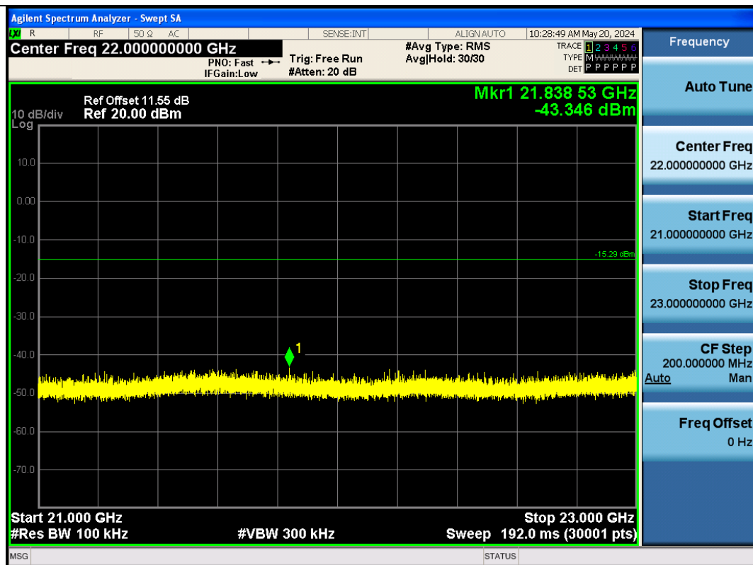
BLE_2M-Ant1-2440-21000~23000-PASS
