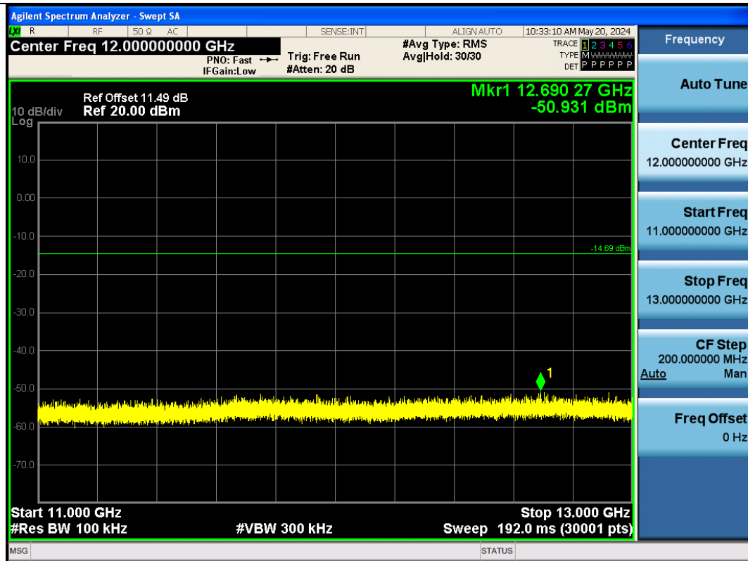
BLE_2M-Ant1-2480-11000~13000-PASS
