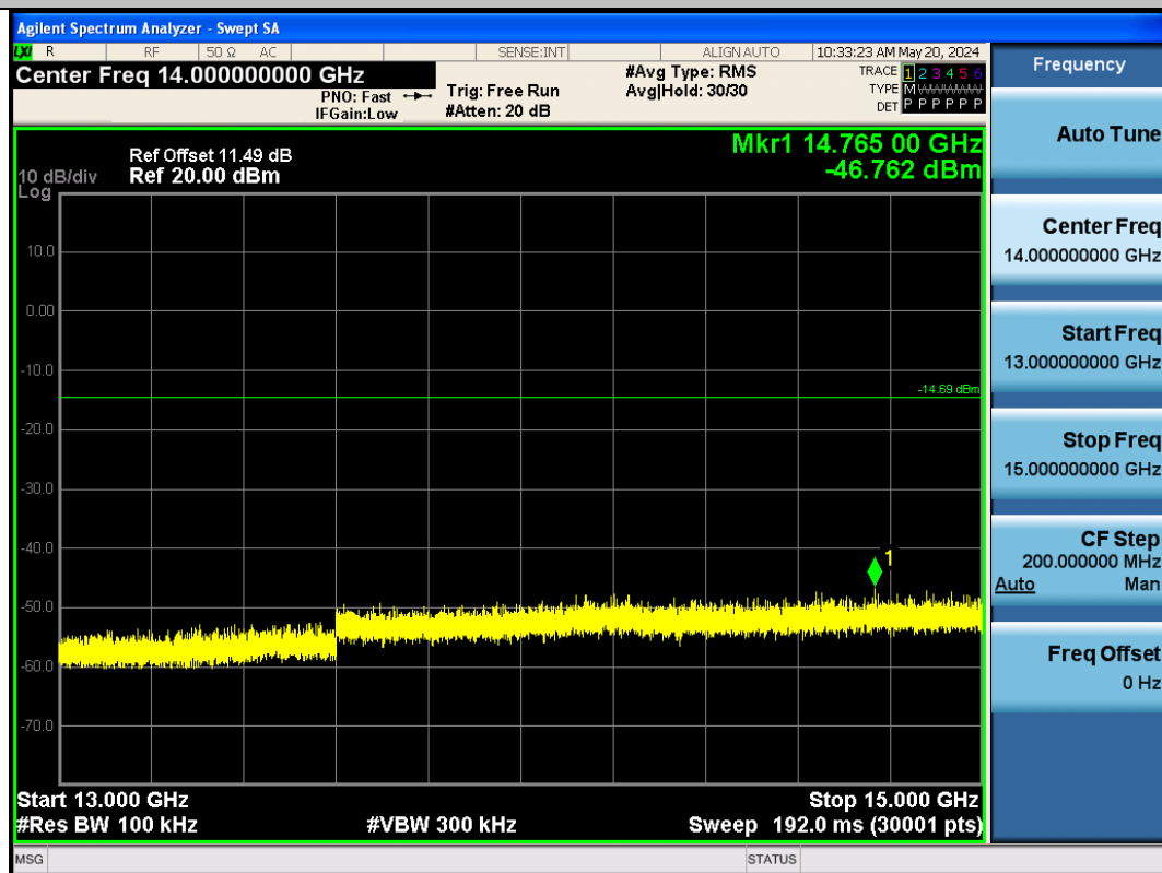
BLE_2M-Ant1-2480-13000~15000-PASS
