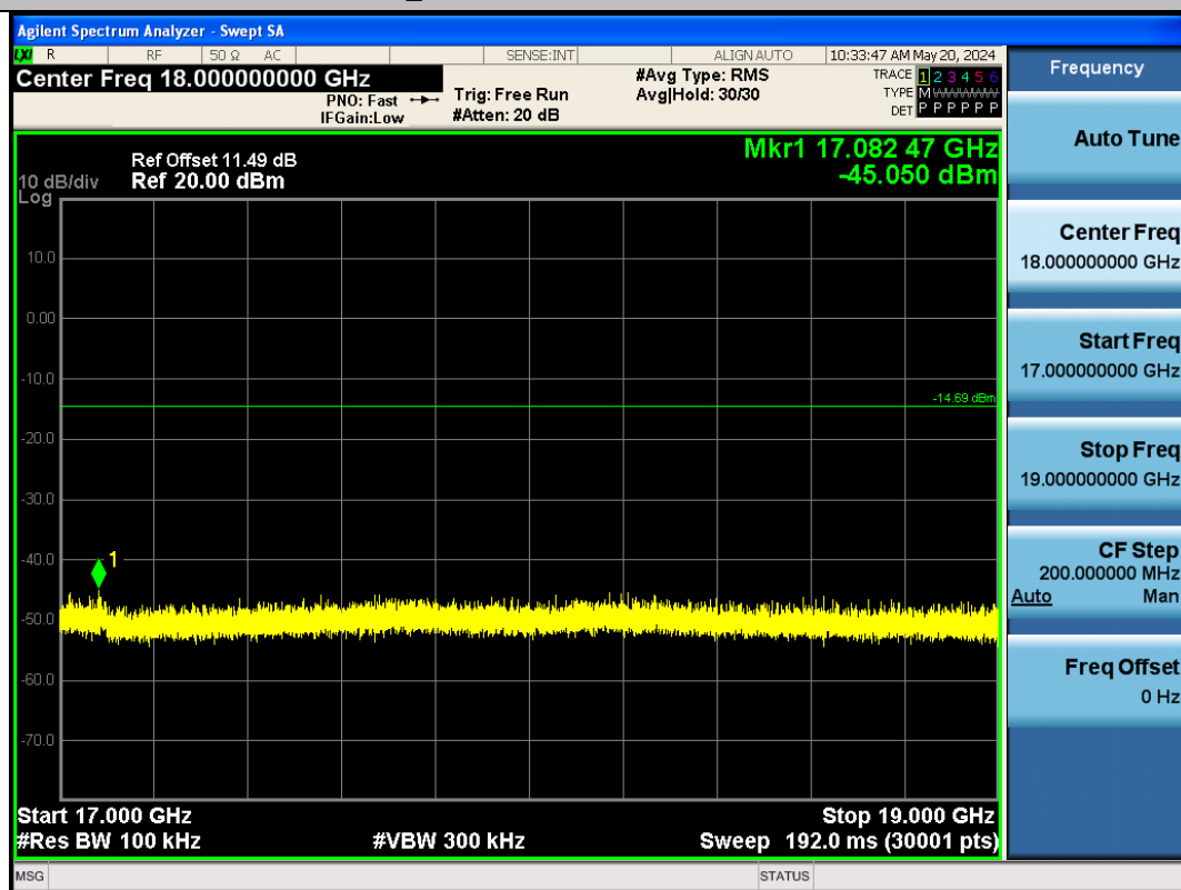
BLE_2M-Ant1-2480-17000~19000-PASS
