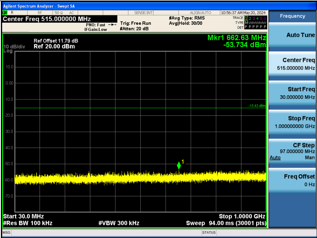
BLE_500K-Ant1-2402-30~1000-PASS
