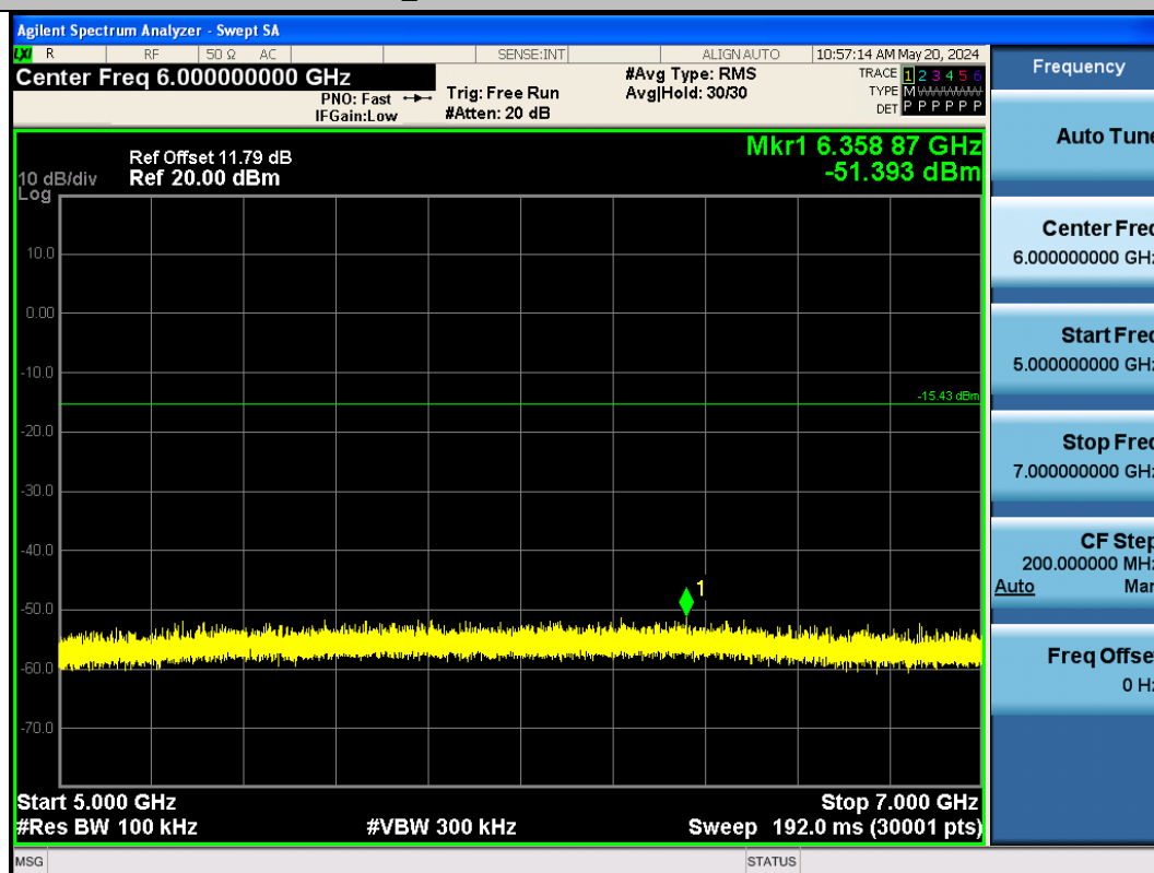
BLE_500K-Ant1-2402-5000~7000-PASS
