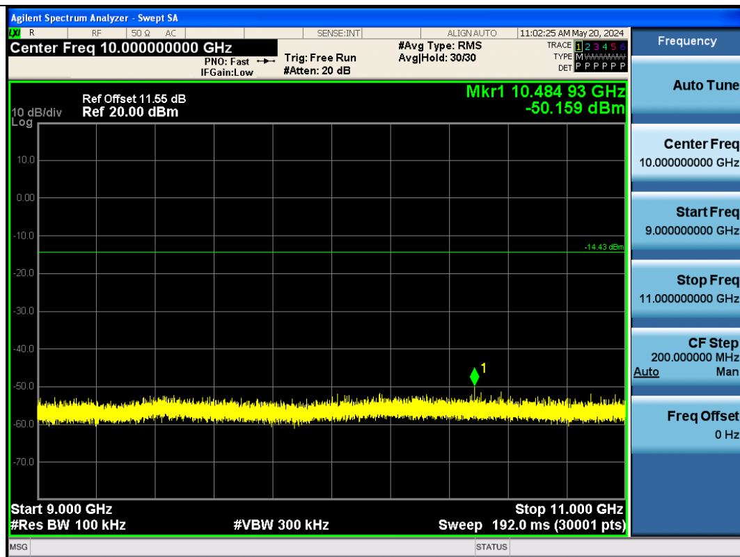
BLE_500K-Ant1-2440-9000~11000-PASS
