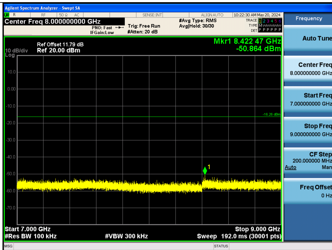
BLE_2M-Ant1-2402-7000~9000-PASS
