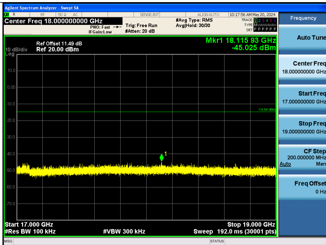
BLE_1M-Ant1-2480-17000~19000-PASS
