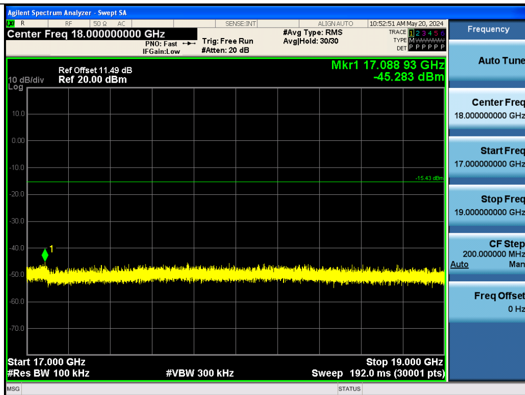
BLE_125K-Ant1-2480-17000~19000-PASS
