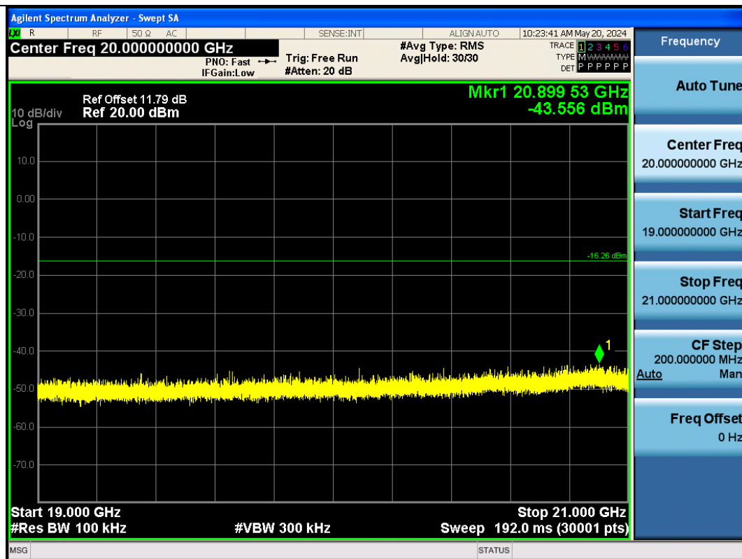
BLE_2M-Ant1-2402-19000~21000-PASS
