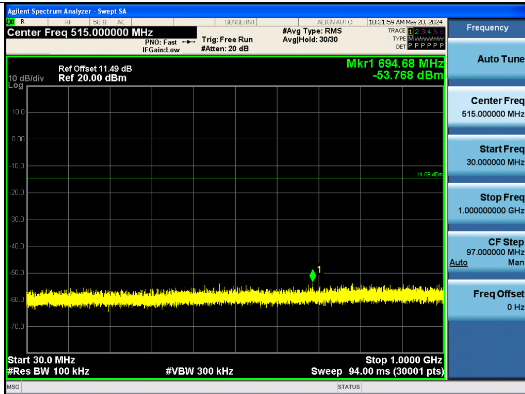
BLE_2M-Ant1-2480-30~1000-PASS
