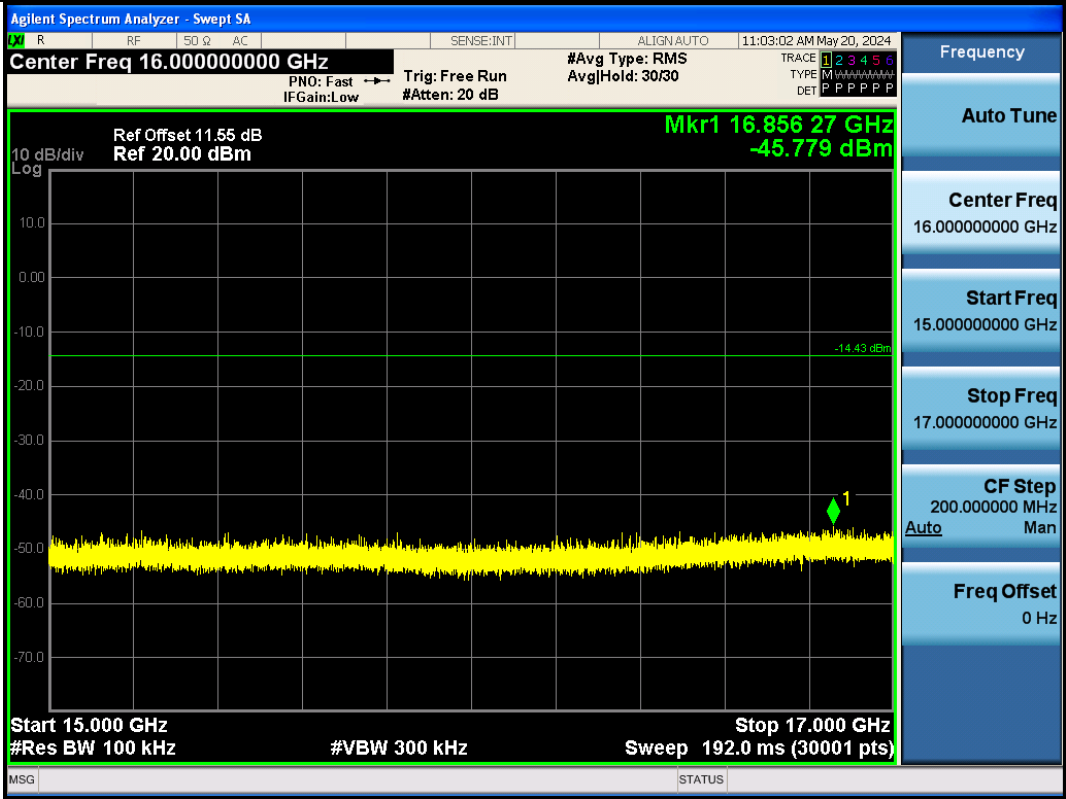
BLE_500K-Ant1-2440-15000~17000-PASS
