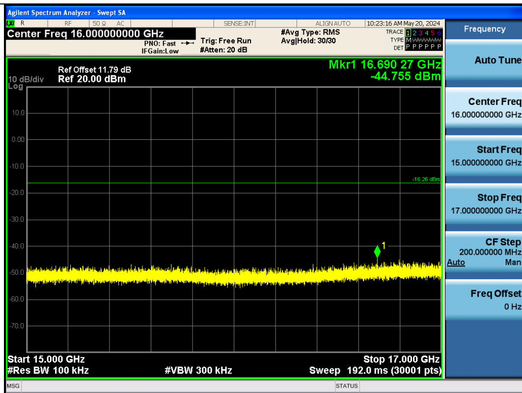
BLE_2M-Ant1-2402-15000~17000-PASS
