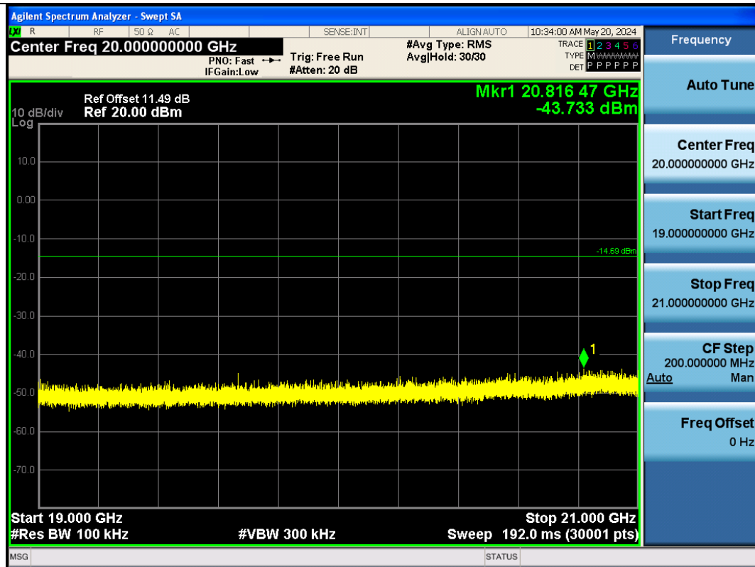
BLE_2M-Ant1-2480-19000~21000-PASS
