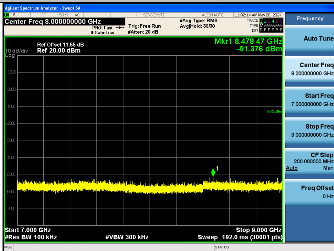
BLE_500K-Ant1-2440-7000~9000-PASS
