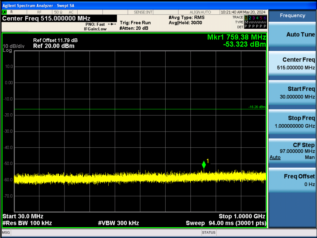
BLE_2M-Ant1-2402-30~1000-PASS
