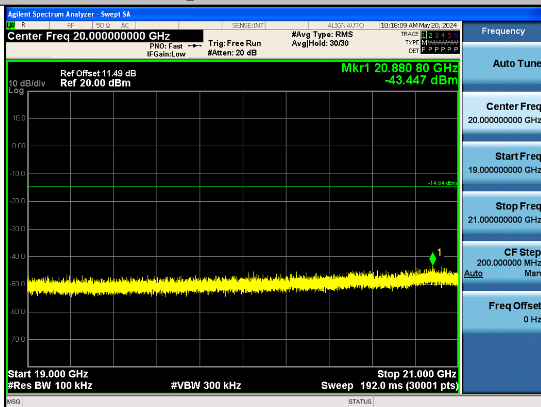
BLE_1M-Ant1-2480-19000~21000-PASS
