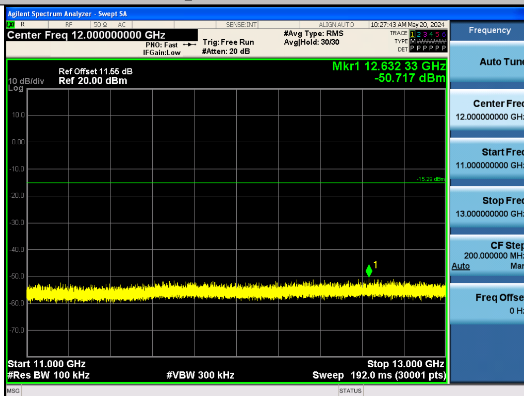
BLE_2M-Ant1-2440-11000~13000-PASS
