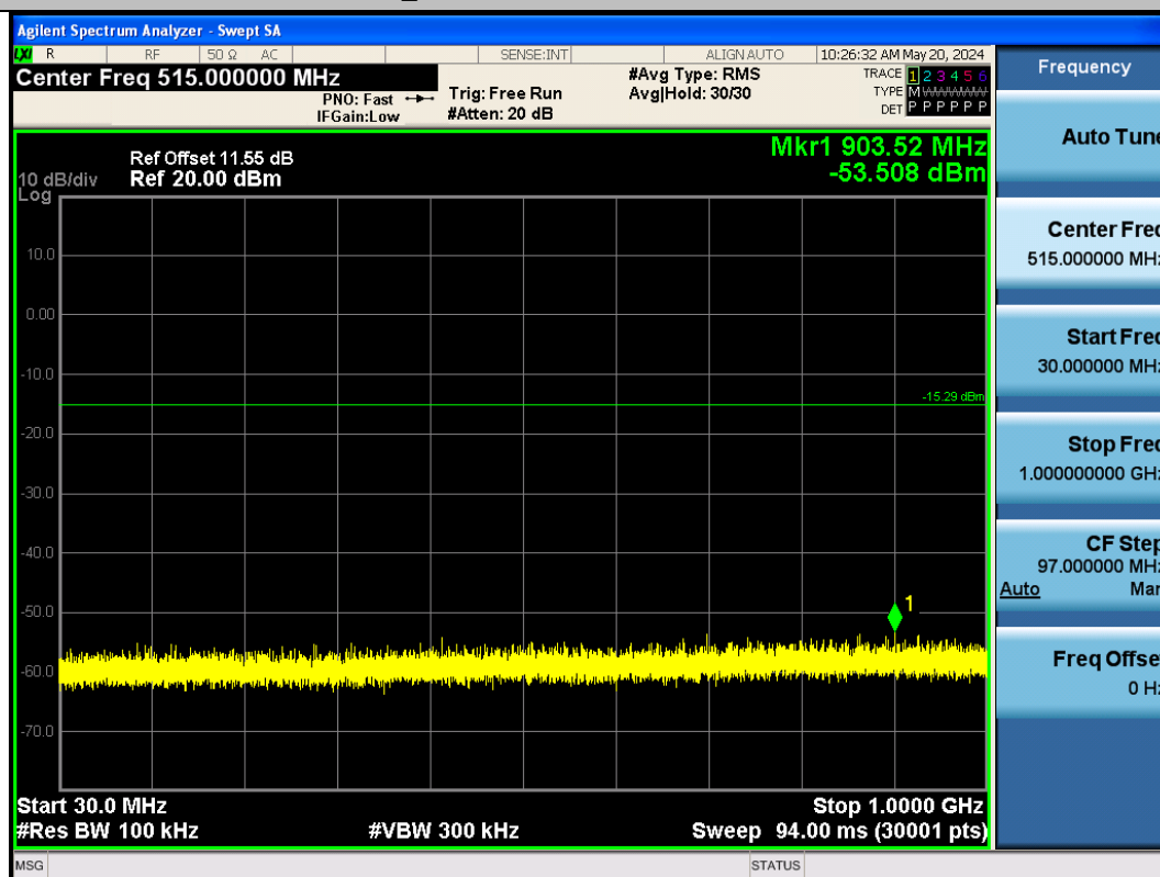
BLE_2M-Ant1-2440-30~1000-PASS
