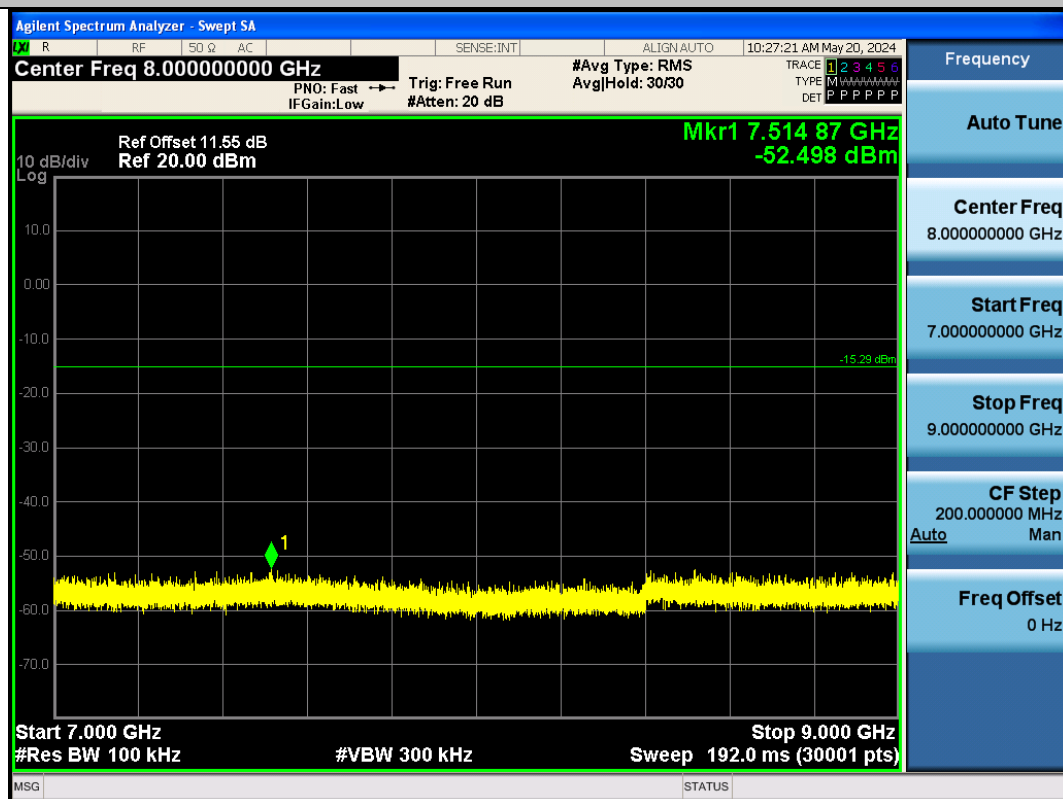
BLE_2M-Ant1-2440-7000~9000-PASS
