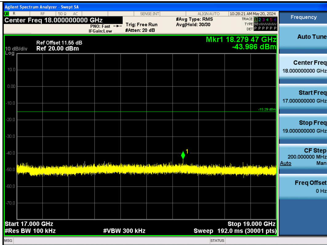
BLE_2M-Ant1-2440-17000~19000-PASS
