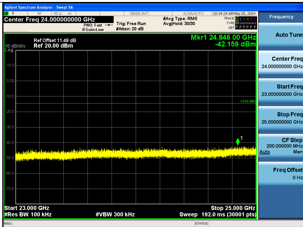
BLE_2M-Ant1-2480-23000~25000-PASS
