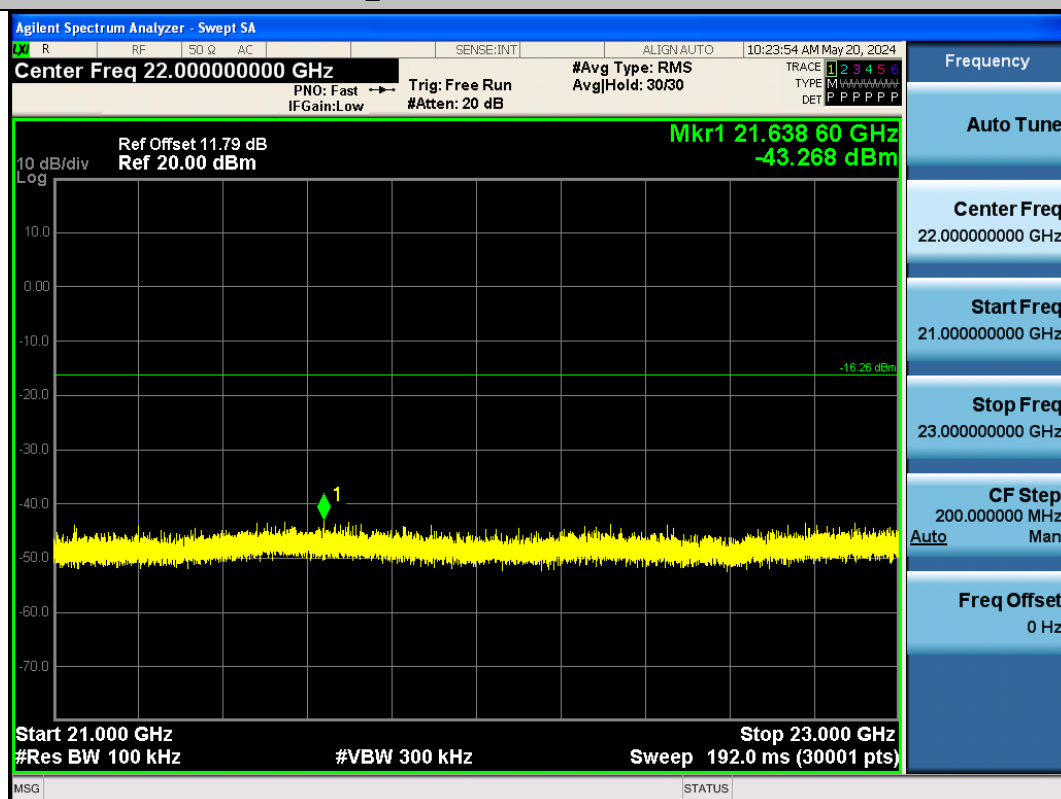
BLE_2M-Ant1-2402-21000~23000-PASS
