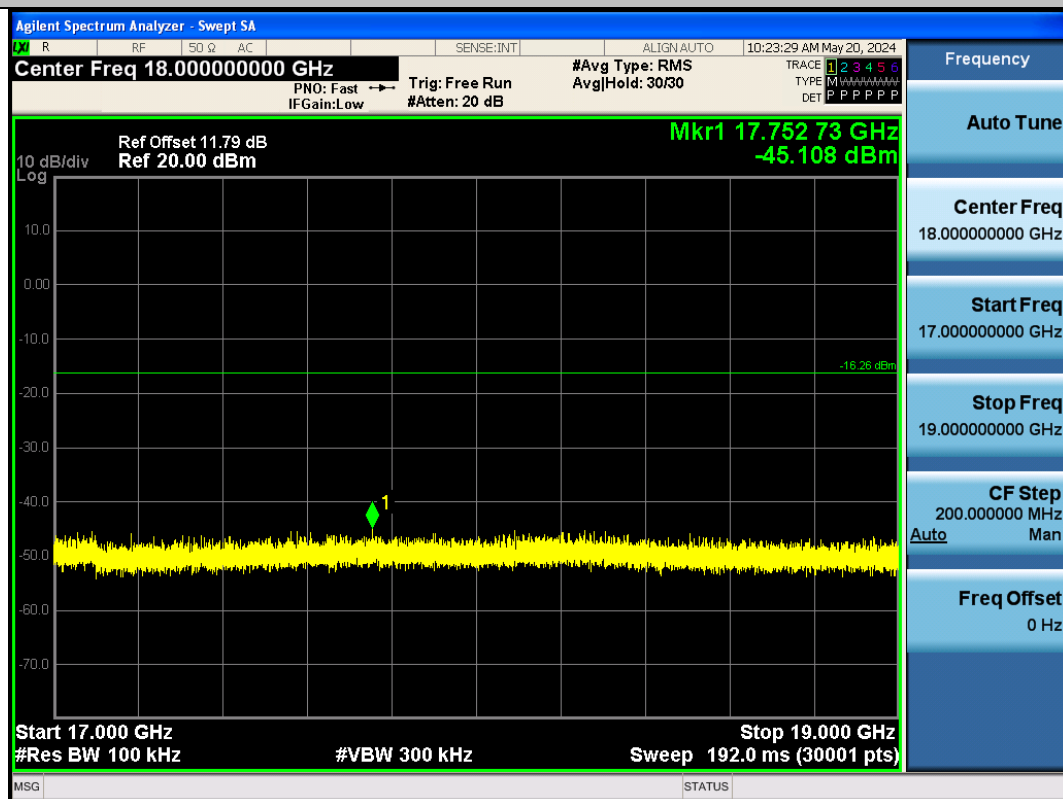
BLE_2M-Ant1-2402-17000~19000-PASS
