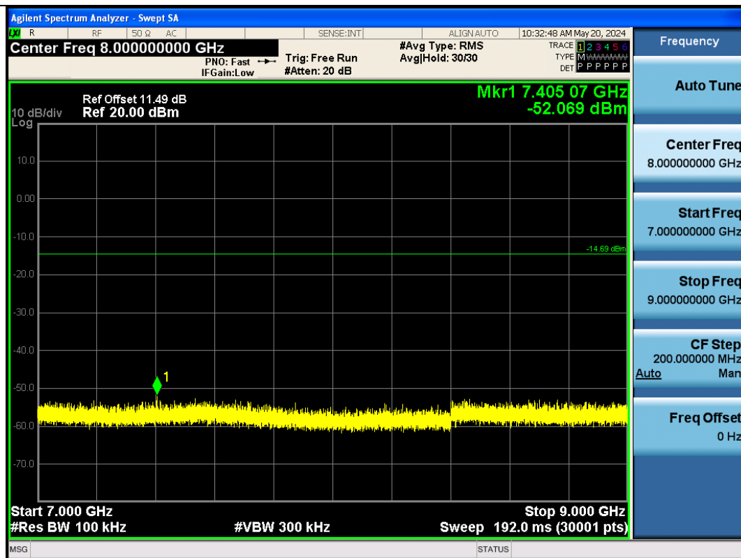
BLE_2M-Ant1-2480-7000~9000-PASS
