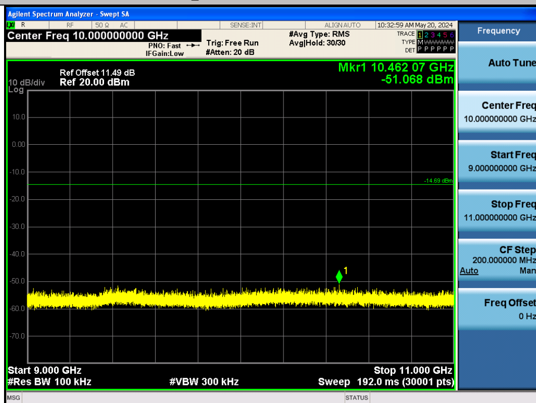
BLE_2M-Ant1-2480-9000~11000-PASS
