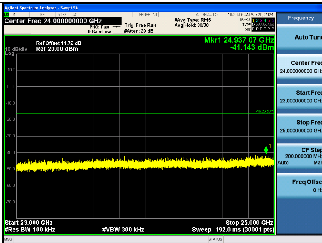
BLE_2M-Ant1-2402-23000~25000-PASS
