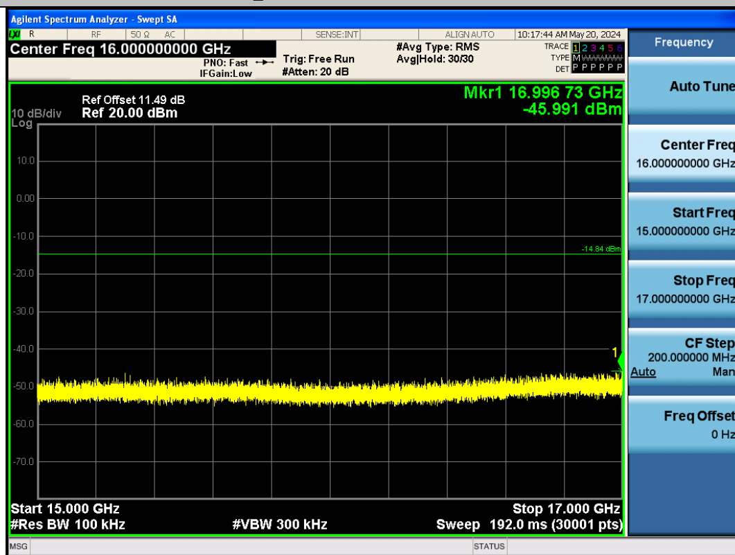
BLE_1M-Ant1-2480-15000~17000-PASS
