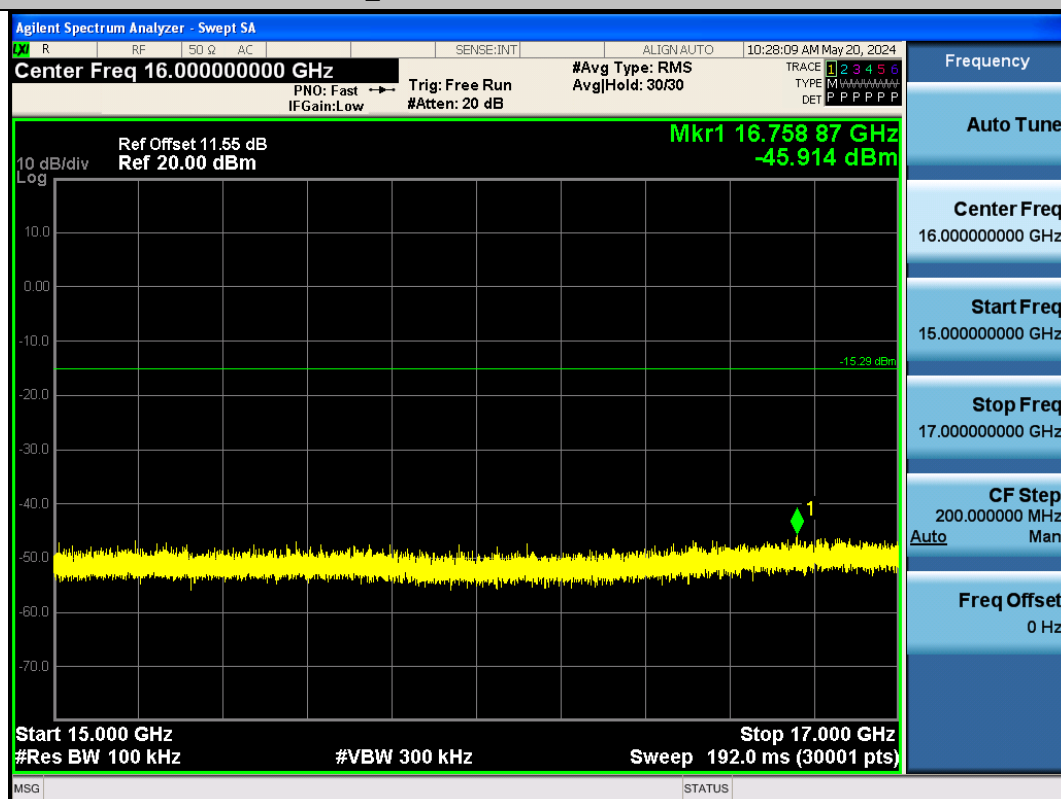
BLE_2M-Ant1-2440-15000~17000-PASS
