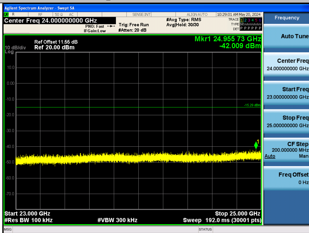
BLE_2M-Ant1-2440-23000~25000-PASS
