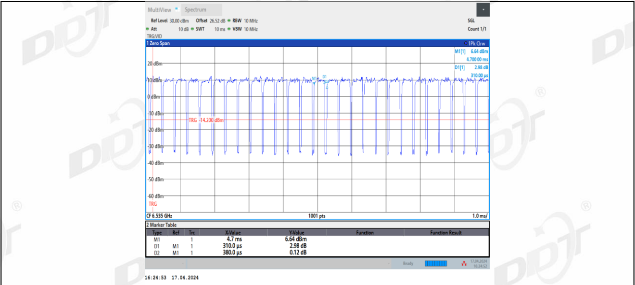
11AX20MIMO_Ant2_6535
