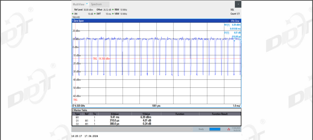
11AX20MIMO_Ant3_6535
