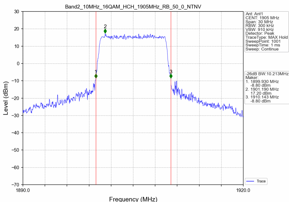
Band2_10MHz_16QAM_HCH_1905MHz_RB_50_0_NTNV
