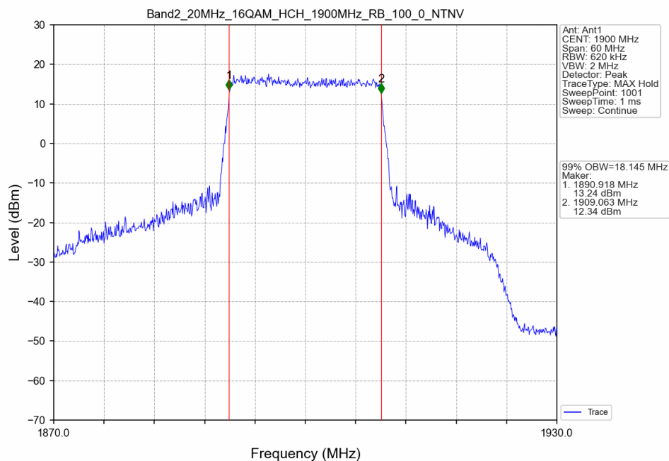
Band2_20MHz_16QAM_HCH_1900MHz_RB_100_0_NTNV
