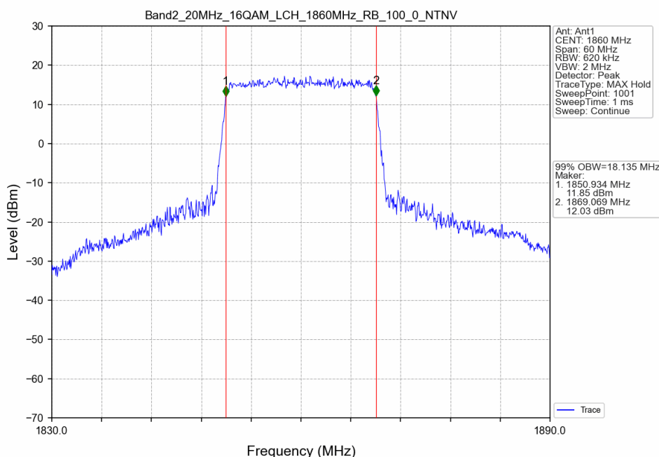
Band2_20MHz_16QAM_LCH_1860MHz_RB_100_0_NTNV
