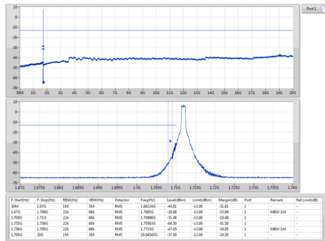
Band 4 LTE-M1_20MHz_Nss1_1TX 1720MHz_16QAM_RB 1,#RB 0,NB 0
