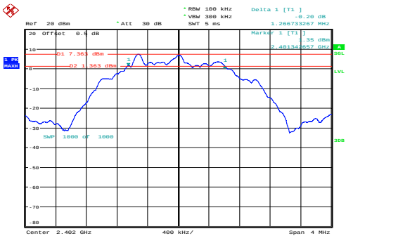
Low 1.267MHz
