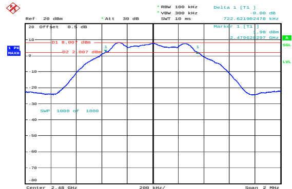
High 0.723MHz
