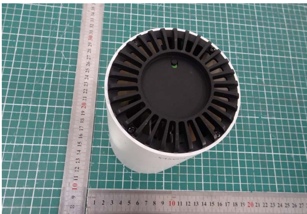
a: EUT
