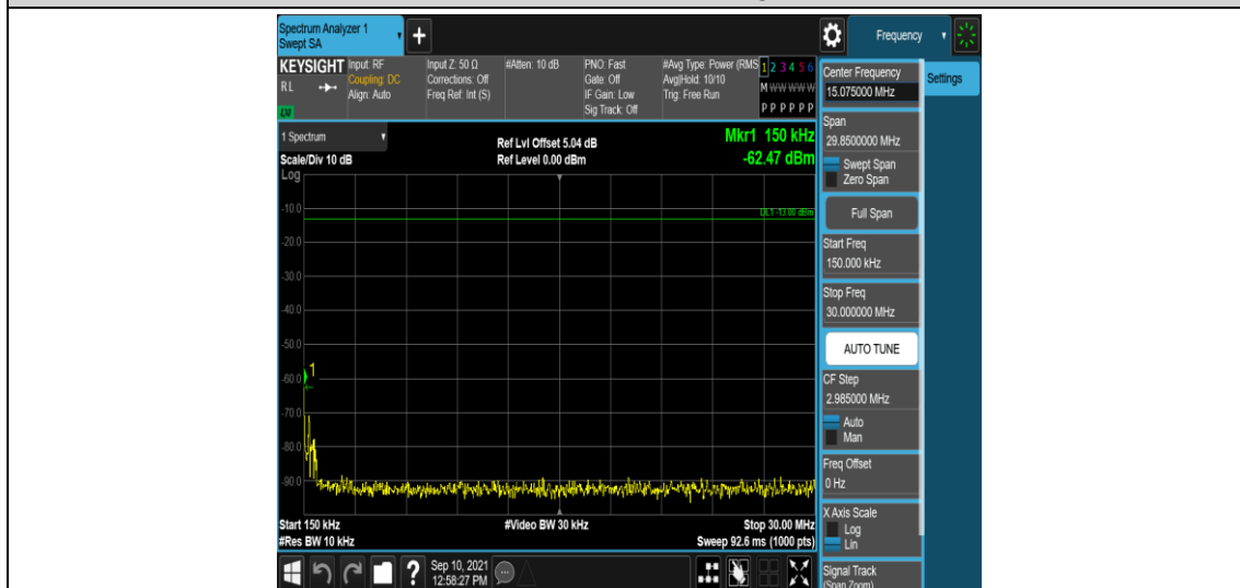
Band5-5MHz-QPSK-20525-1RB#0-Range2:0.15~30MHz
