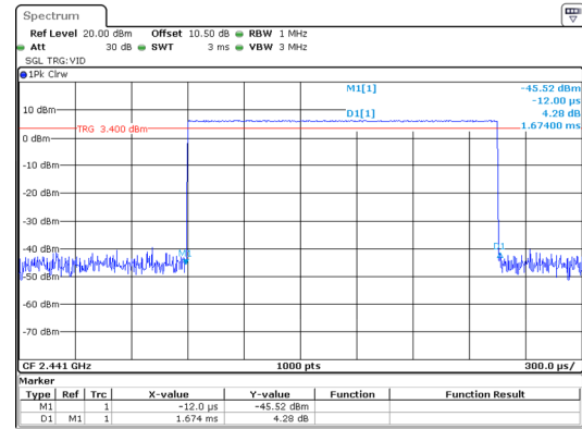
GFSK_Hopping_DH3 1.674ms
