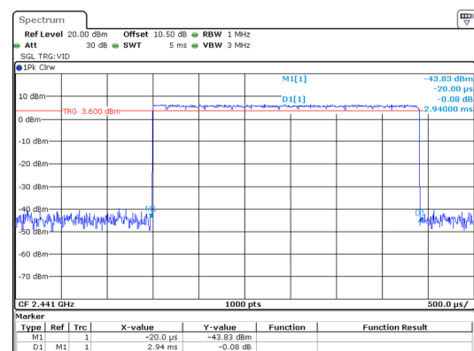
\pi/4 -DQPSK_Hopping_2DH5 2.940ms
