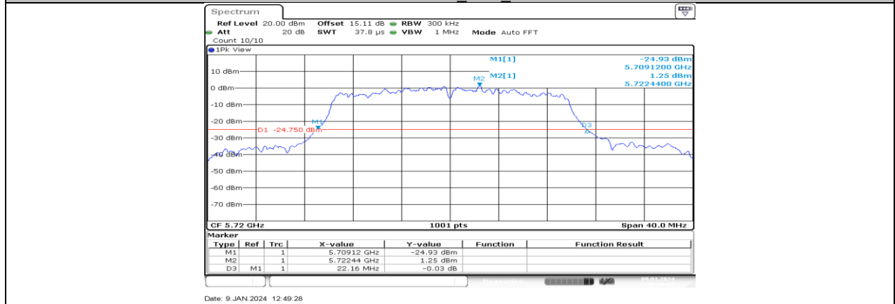
11AX20MIMO_Ant2_5720
