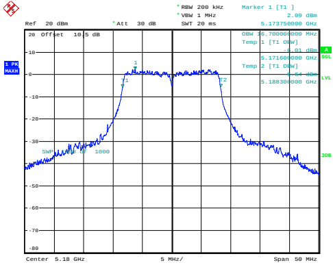
a_5180MHz_Chain 0 16.700MHz
