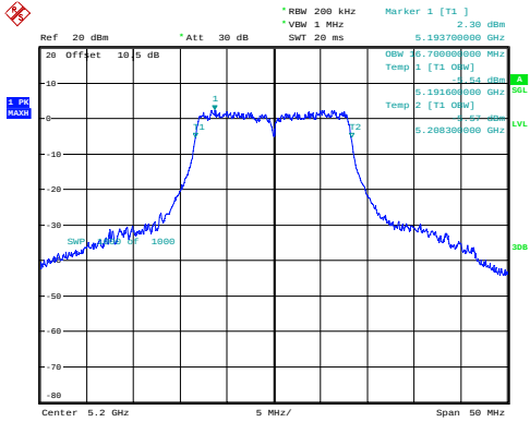
a_5200MHz_Chain 0 16.700MHz
