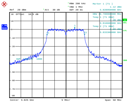
a_5825MHz_Chain 0 16.700MHz
