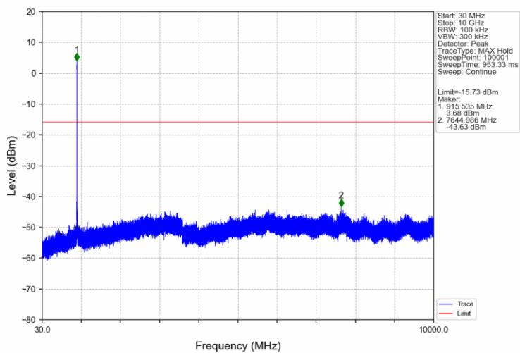
BW 2M_MCH_915MHz_Ant1_NTNV
