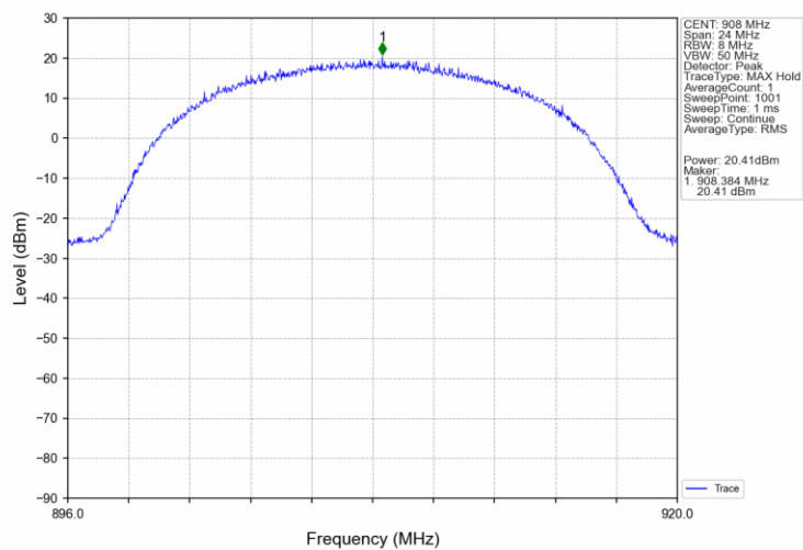
BW 8M_LCH_908MHz_Ant1_NTNV
