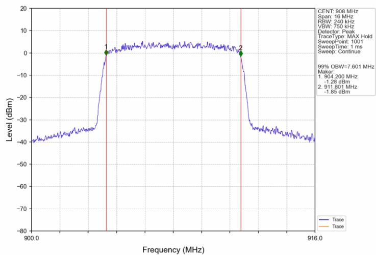
BW 8M_LCH_908MHz_Ant1_NTNV
