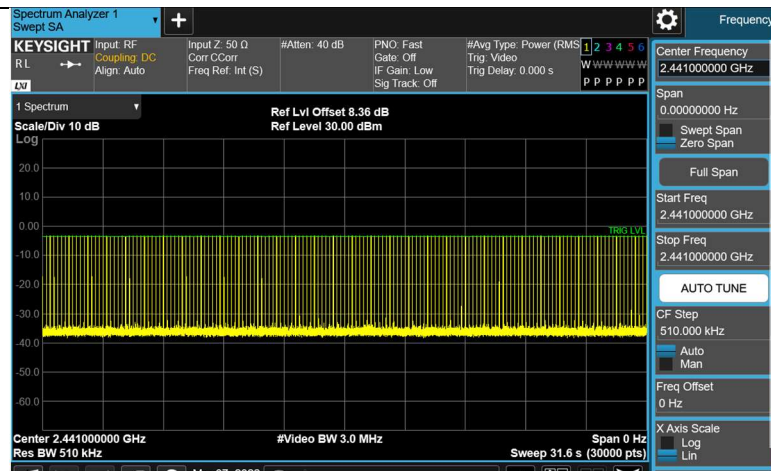
3DH5_Ant1_Hop
