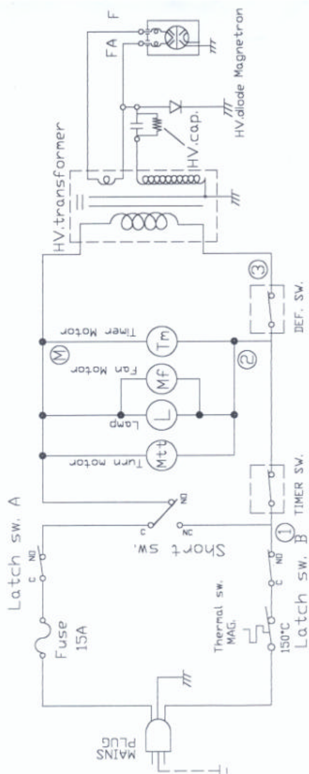
TMO-1960M WIRING DIAGRAM
