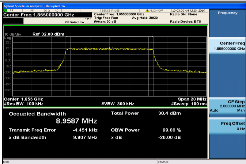
Band2-10MHz-QPSK-18650-50RB#0-8.9587
