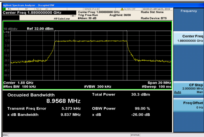
Band2-10MHz-QPSK-18900-50RB#0-8.9568
