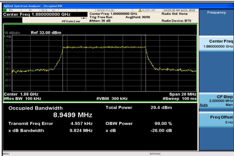
Band2-10MHz-16QAM-18900-50RB#0-8.9499
