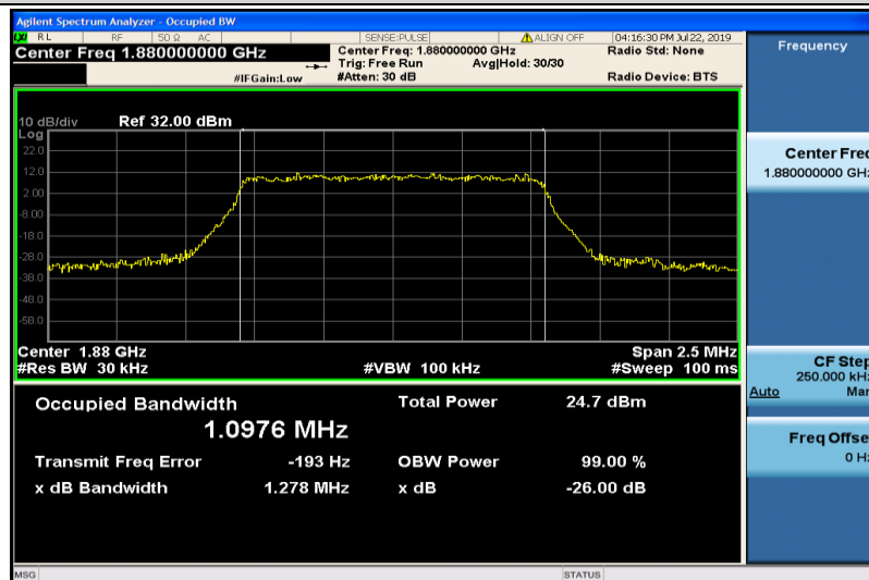
Band2-1.4MHz-QPSK-18900-6RB#0-1.0976
