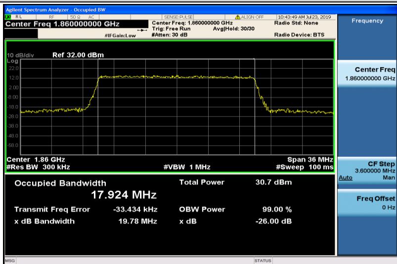
Band2-20MHz-QPSK-18700-100RB#0-17.924
