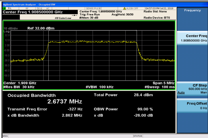
Band2-3MHz-QPSK-19185-15RB#0-2.6737
