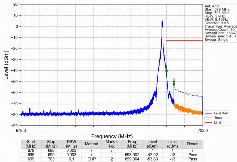
n71_15kHz_SISO_NTNV_20MHz_DFT-s-OFDM PI/2 BPSK_688MHz_Edge_1RB_Right
