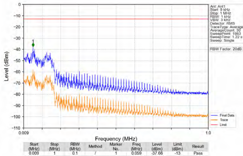
n71_15kHz_SISO_NTNV_20MHz_DFT-s-OFDM PI/2 BPSK_688MHz_Edge_1RB_Right
