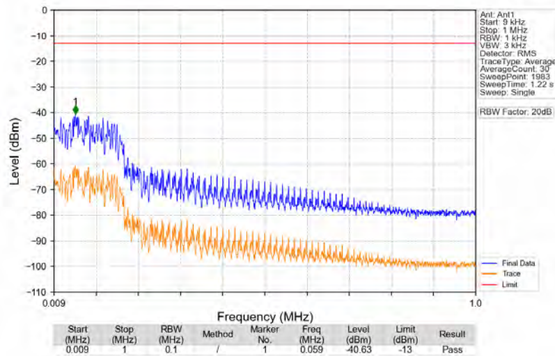
n71_15kHz_SISO_NTNV_20MHz_DFT-s-OFDM_QPSK_688MHz_Edge_1RB_Right
