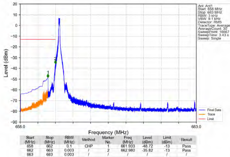
n71_15kHz_SISO_NTNV_20MHz_DFT-s-OFDM PI/2 BPSK_673MHz_Edge_1RB_Left
