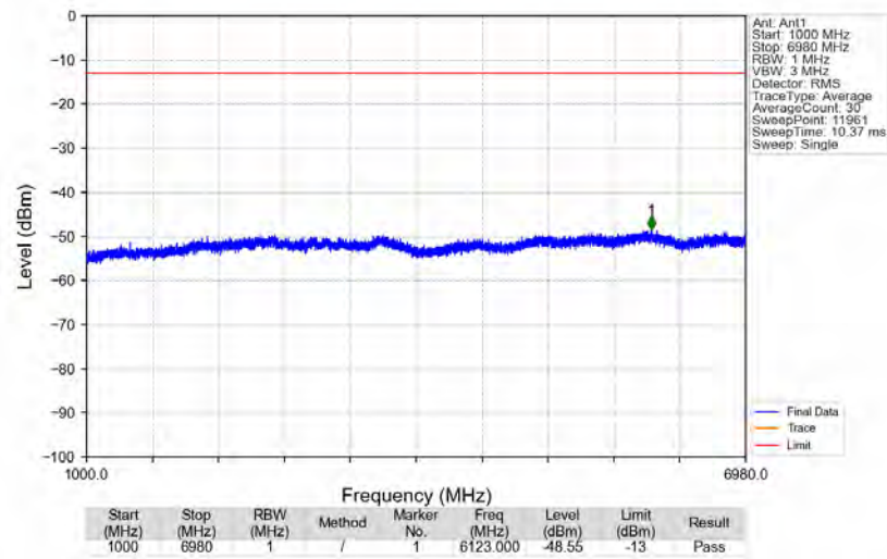
n71_15kHz_SISO_NTNV_20MHz_DFT-s-OFDM_PI/2_BPSK_688MHz_Edge_1RB_Right
