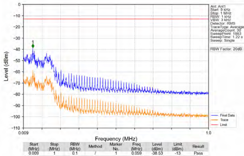
n71_15kHz_SISO_NTNV_20MHz_DFT-s-OFDM PI/2 BPSK_673MHz_Edge_1RB_Left
