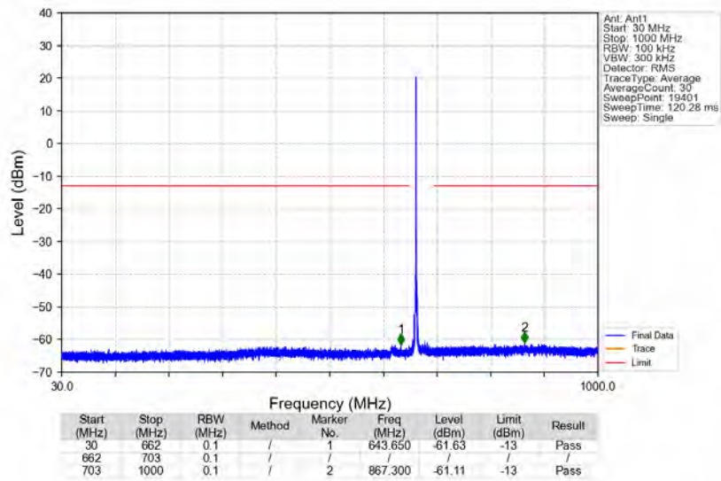
n71_15kHz_SISO_NTNV_20MHz_DFT-s-OFDM_PI/2_BPSK_680.5MHz_Edge_1RB_Left
