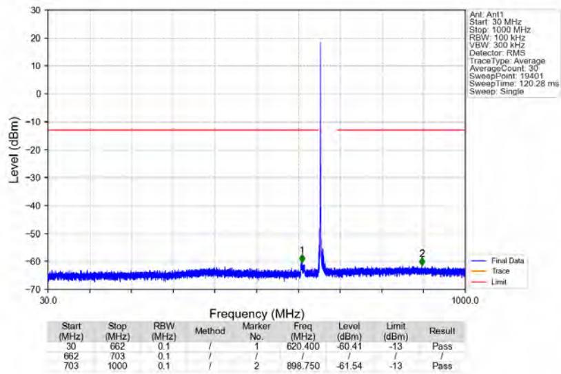
n71_15kHz_SISO_NTNV_10MHz_DFT-s-OFDM_PI/2_BPSK_668MHz_Edge_1RB_Left
