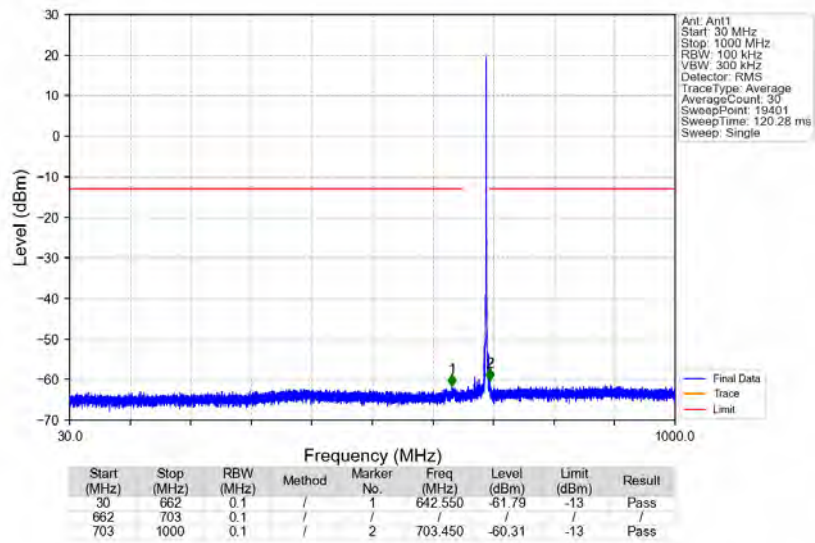
n71_15kHz_SISO_NTNV_20MHz_DFT-s-OFDM PI/2 BPSK_688MHz_Edge_1RB_Right
