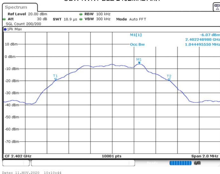
OBW NVNT BLE 2402MHz Ant1
