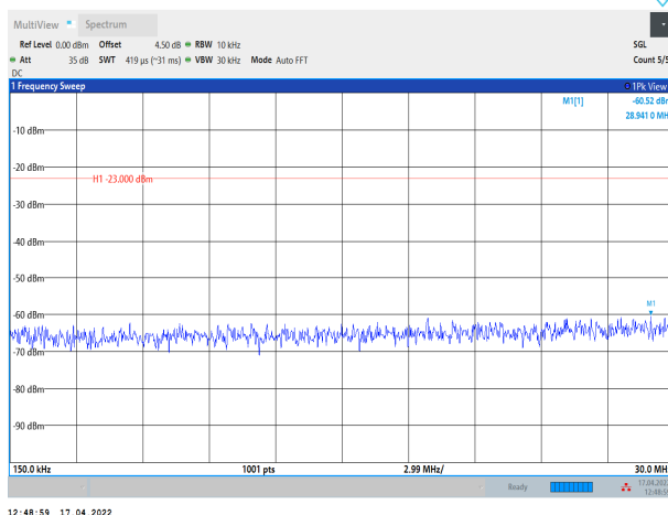
Band71-20MHz-QPSK-133222-1RB#0-Range2:0.15~30MHz
