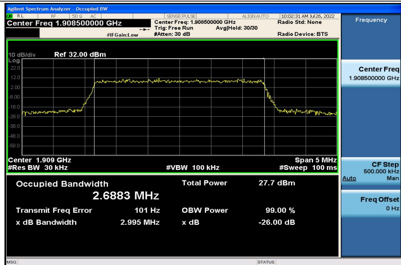
Band2-3MHz-QPSK-19185-15RB#0-2.6883
