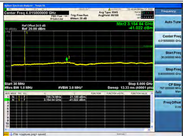
Band14 / 10MHz / Low CH / 64QAM
