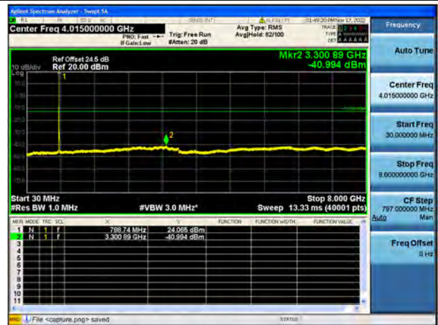
Band14 / 10MHz / Low CH / QPSK
