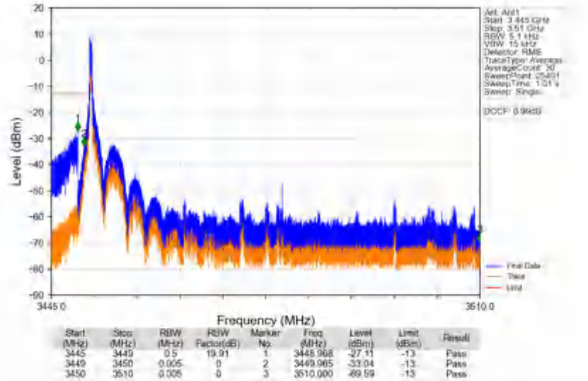
n78e_30kHz_SISO_NTNV_60MHz_DFT-s-OFDM_PI/2_BPSK_3480MHz_Edge_1RB_Left
