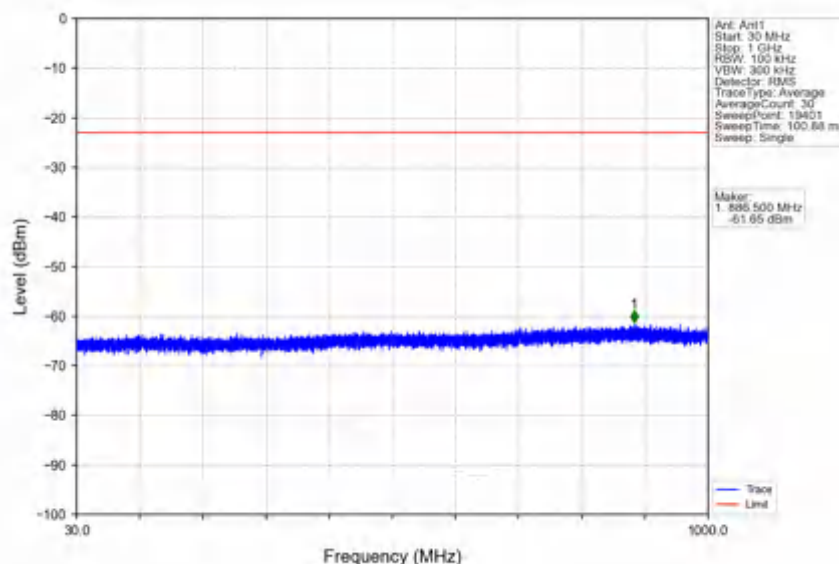
n78e_30kHz_SISO_NTV_90MHz_CP-OFDM QPSK_3495MHz_Inner_1RB_Left
