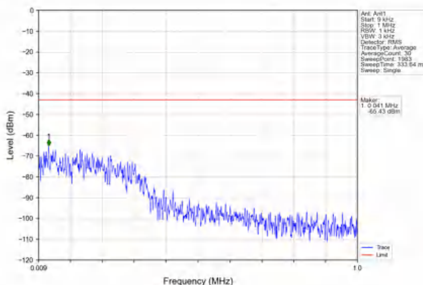
n78e 30kHz SISO NTNV 60MHz CP-OFDM QPSK 3519.99MHz Edge 1RB Right
