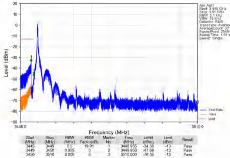
n78e_30kHz_SISO_NTNV_60MHz_DFT-s-OFDM_PI/2_BPSK_3480MHz_Inner_1RB_Left
