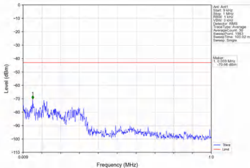
n78e_30kHz_SISO_NTNV_90MHz_DFT-s-OFDM PI/2 BPSK_3495MHz_Inner_1RB_Left
