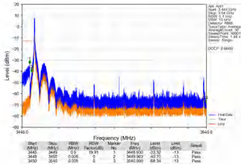
n78e_30kHz_SISO_NTNV_90MHz_DFT-s-OFDM PI/2 BPSK_3495MHz_Inner_1RB_Left
