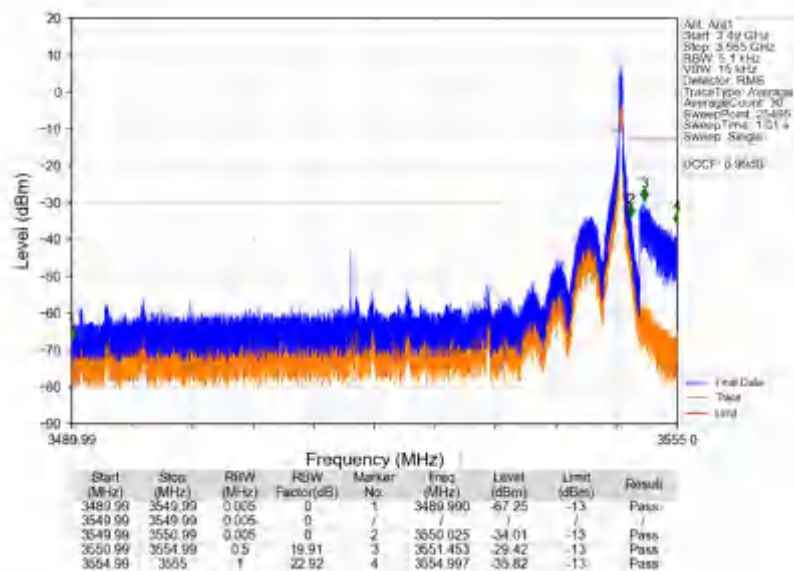
n78e 30kHz SISO NTNV 60MHz CP-OFDM QPSK 3519.99MHz Edge 1RB Right
