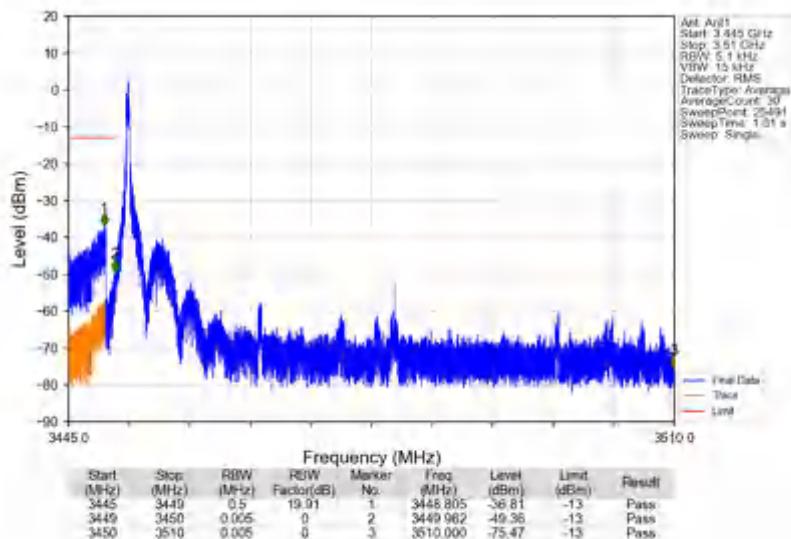
n78e_30kHz_SISO_NTNV_60MHz_DFT-s-OFDM_QPSK_3480MHz_Inner_1RB_Left
