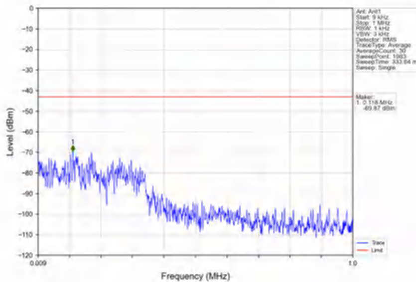
n78e_30kHz_SISO_NTNV_60MHz_DFT-s-OFDM_PI/2_BPSK_3480MHz_Edge_1RB_Left
