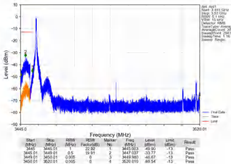
n78e_30kHz_SISO_NTNV_70MHz_DFT-s-OFDM_QPSK_3485.01MHz_Inner_1RB_Left
