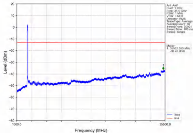
n78e_30kHz_SISO_NTNV_90MHz_DFT-s-OFDM QPSK_3495MHz_Inner_1RB_Left
