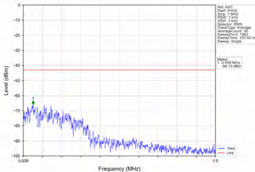
n78e_30kHz_SISO_NTV_60MHz_CP-OFDM QPSK_3480MHz_Inner_1RB_Left
