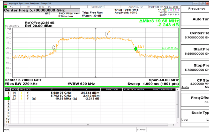
11N20MIMO_Ant1_5700
