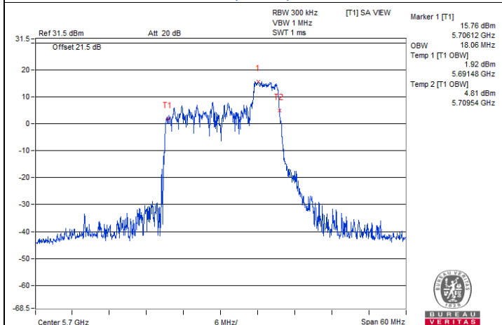
802.11ax (HE20) 52-tone RU : CH 140@40
