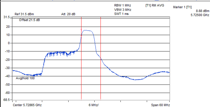
802.11ax (HE20) 26-tone RU : CH 144@8 (U-NII-3)
