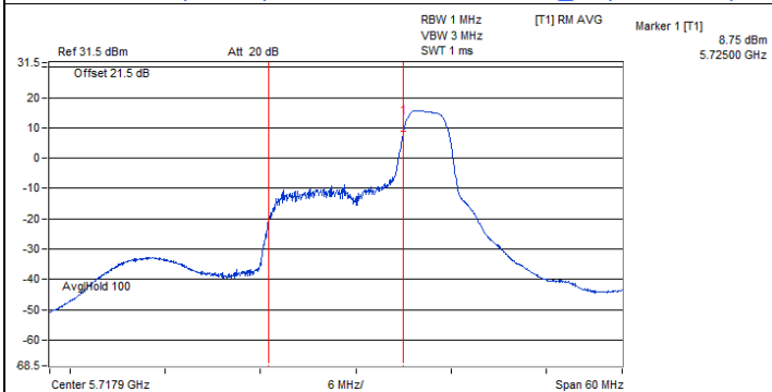
802.11ax (HE20) 26-tone RU : CH 144@8 (U-NII-2C)
