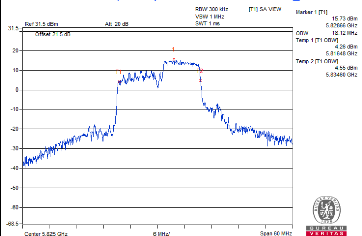
802.11ax (HE20) 106-tone RU : CH 165@54
