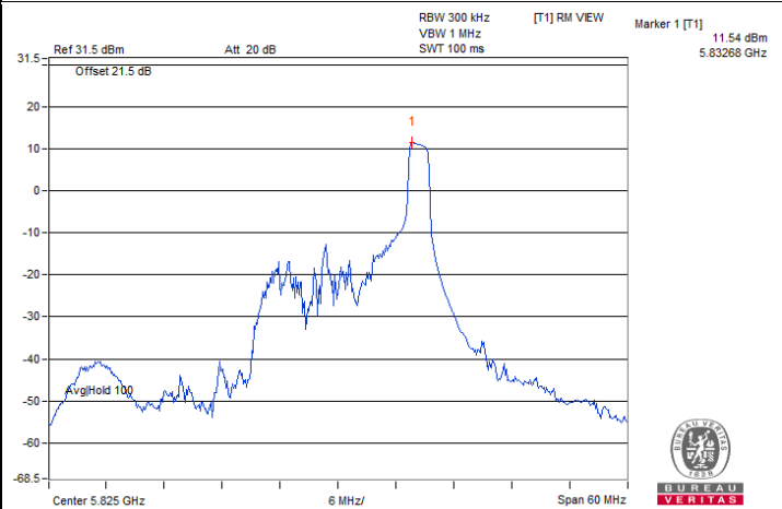
802.11ax (HE20) 26-tone RU : CH 165@8
