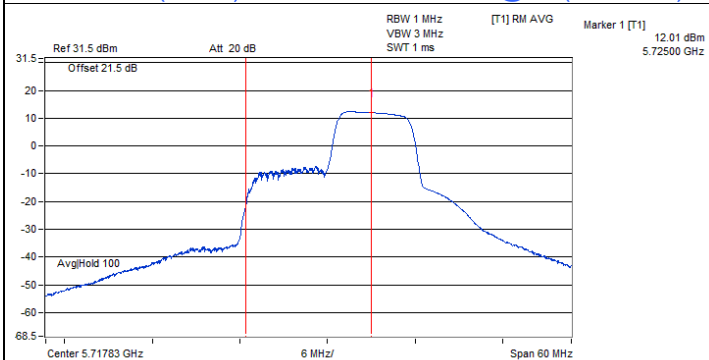
802.11ax (HE20) 52-tone RU : CH 144@40 (U-NII-2C)
