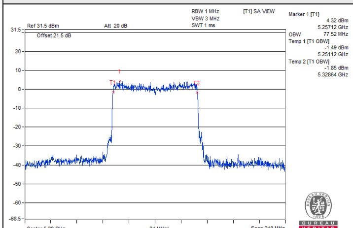
802.11ax (HE80) : CH 58
