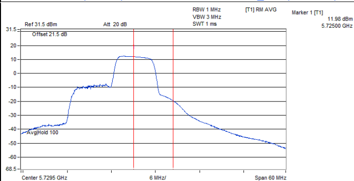
802.11ax (HE20) 52-tone RU : CH 144@40 (U-NII-3)
