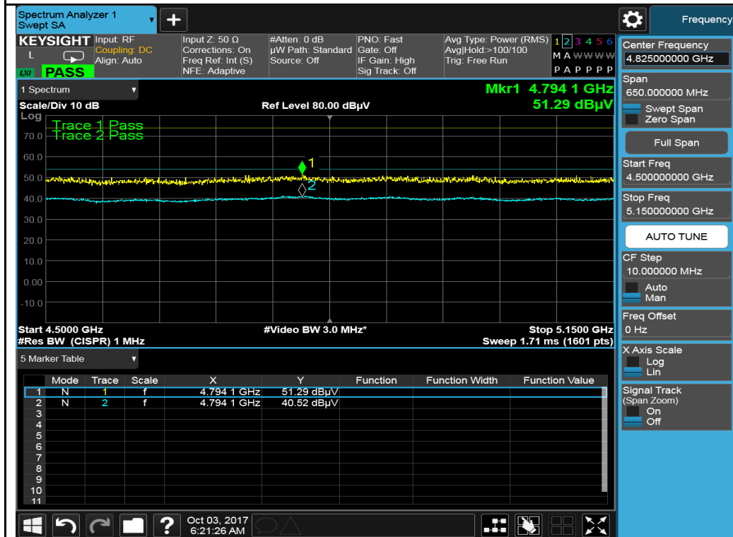
802.11ac-VHT80 5210MHz
