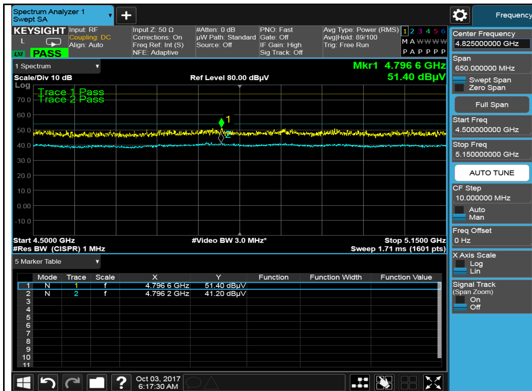
802.11n-HT40 5190MHz
