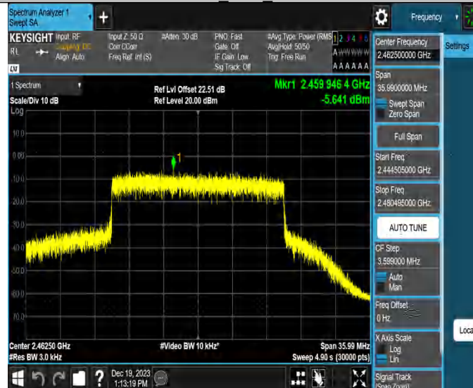
20MHz Ant1 2462.5
