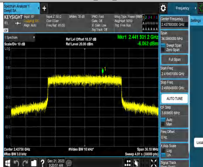
20MHz_Ant0_2437.5
