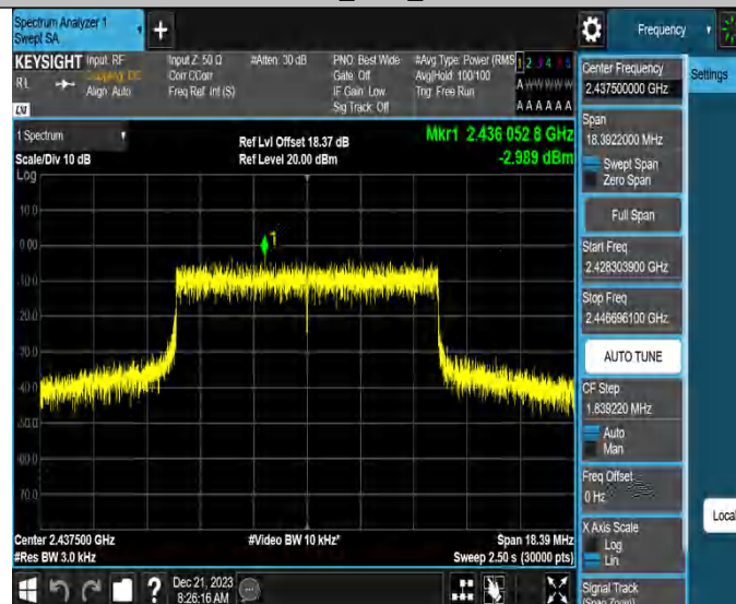
10MHz_Ant0_2437.5
