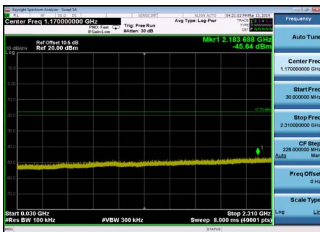
,Plot 3,30MHz~2310MHz-802.11g,2437MHz
