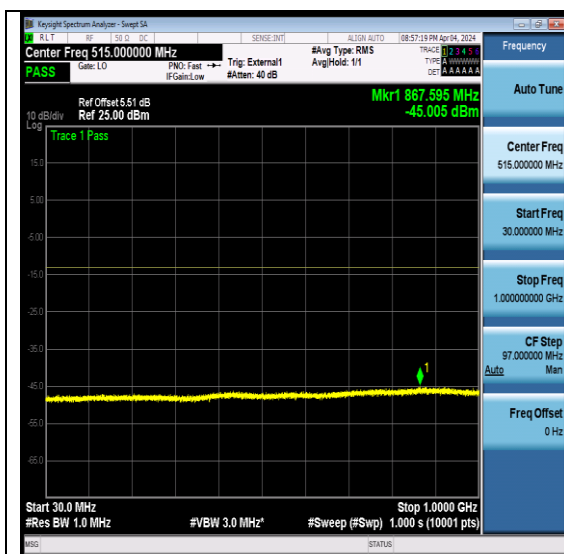
NTNV-N78-3450-3550-PC2-30-20-H-CP- QPSK-Edge_1RB_Left-Ant7-PASS
