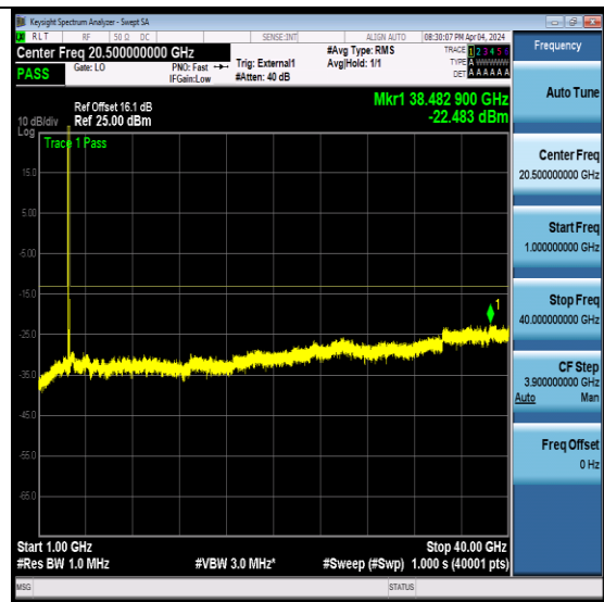
NTNV-N78-3450-3550-PC2-30-100-M-CP-QPSK- Edge_1RB_Left-Ant7-PASS
