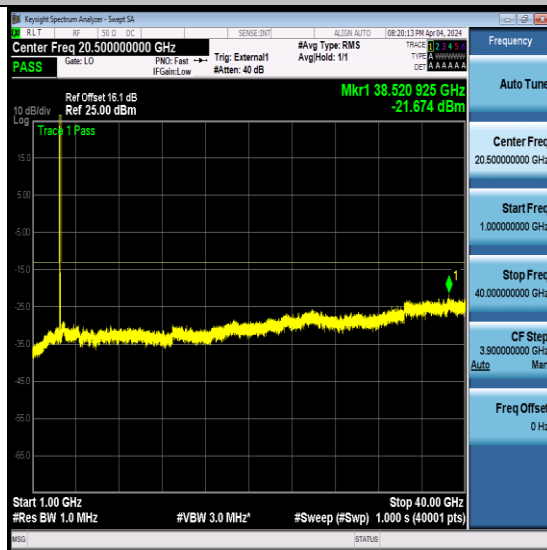
NTNV-N78-3450-3550-PC2-30-60-L-CP-QPSK- Edge_1RB_Left-Ant7-PASS
