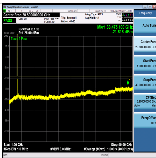
NTNV-N78-3450-3550-PC2-30-20-H-CP- QPSK-Edge_1RB_Left-Ant7-PASS
