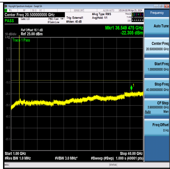
NTNV-N78-3450-3550-PC2-30-20-M-CP-QPSK- Edge_1RB_Left-Ant1-PASS
