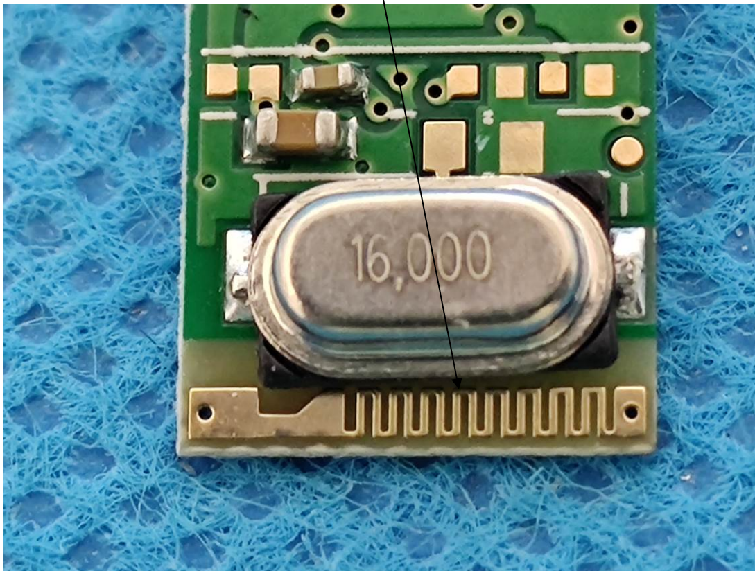
Antenna
