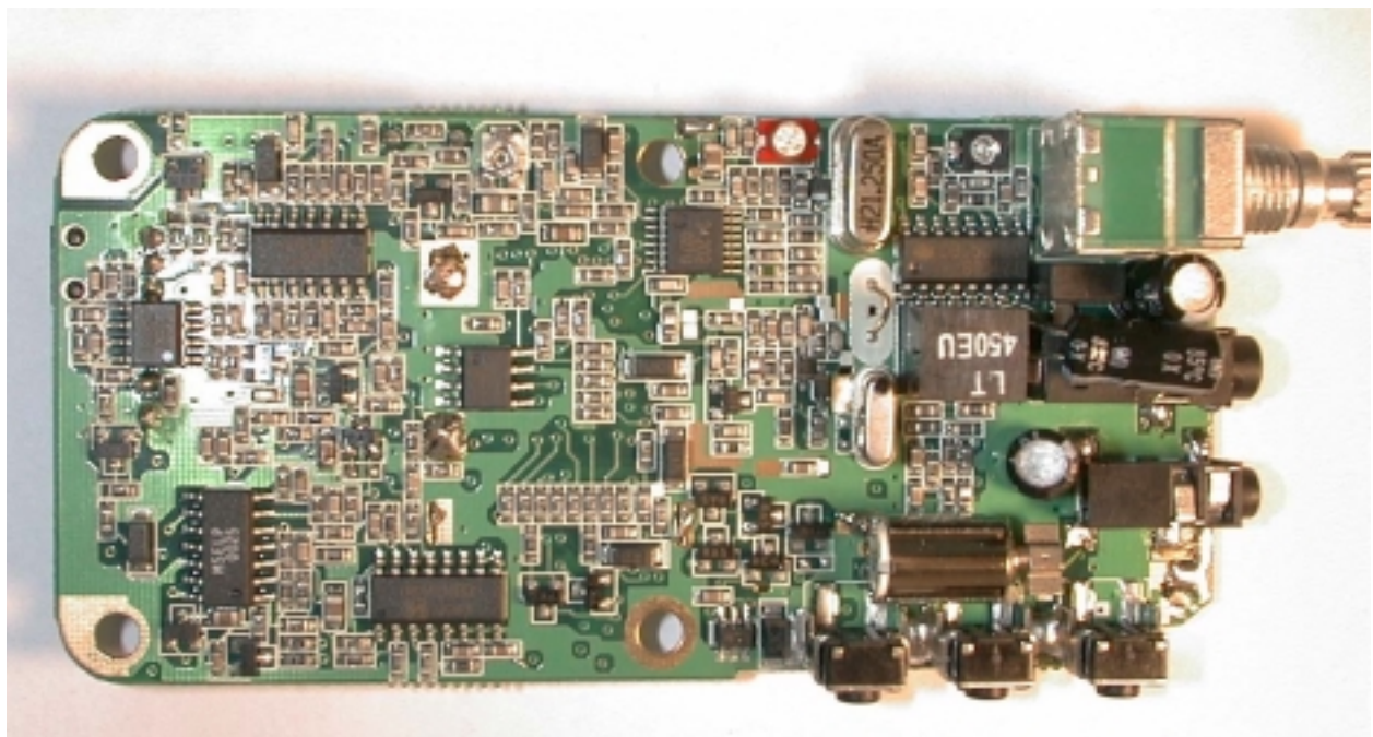
Bottom PCB
