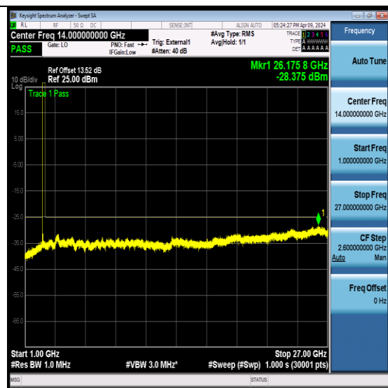
NTN-N41-PC2-30-60-L-CP-QPSK- Edge_1RB_Left-Ant0-PASS
