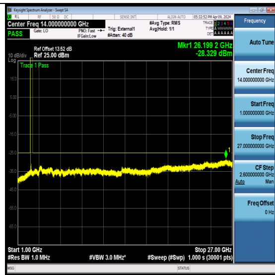
NTVN-N41-PC2-30-100-M-CP-QPSK- Edge_1RB_Left-Ant0-PASS
