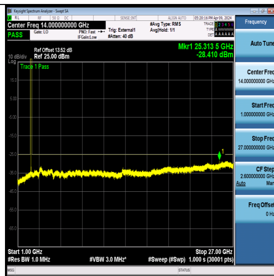
NTNV-N41-PC2-30-20-M-CP-QPSK- Edge_1RB_Left-Ant0-PASS
