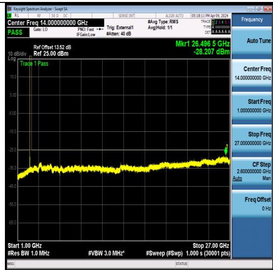
NTVN-N41-PC2-30-20-L-CP-QPSK- Edge_1RB_Left-Ant0-PASS
