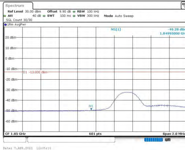
Band2-5MHz-QPSK-18625-1RB#24
