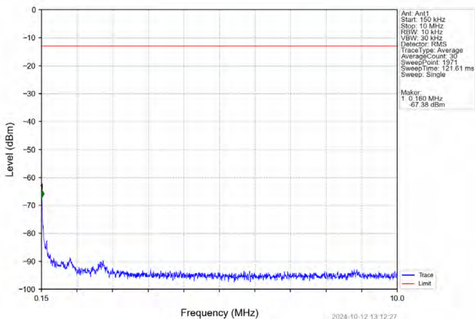
Band66_10MHz_QPSK_HCH_1775MHz_RB_1_0 NTNV
