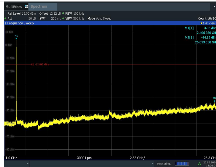
11BE20MIMO_Ant0_2412_52Tone_RU40_0~Reference
