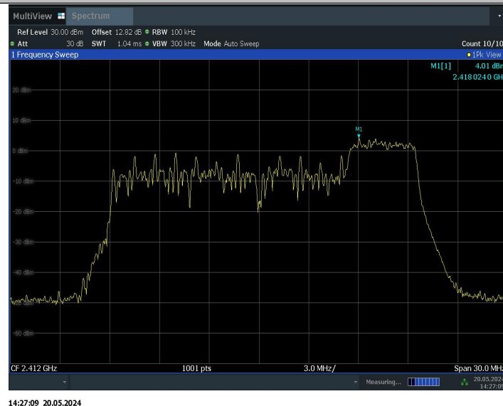
11BE20MIMO_Ant0_2412_52Tone_RU40_30~1000
