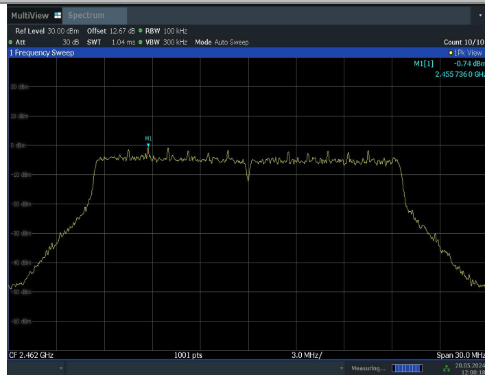
11AX20MIMO_Ant0_2462_0~Reference
