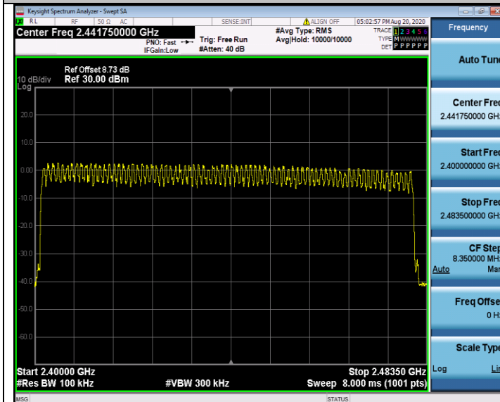
8DPSK
