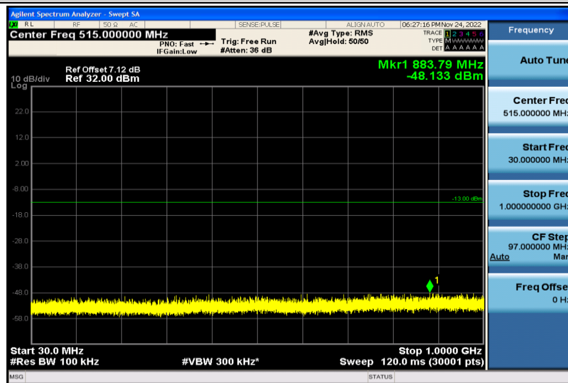
Band4-20MHz-QPSK-20050-1RB#0-30~1000MHz
