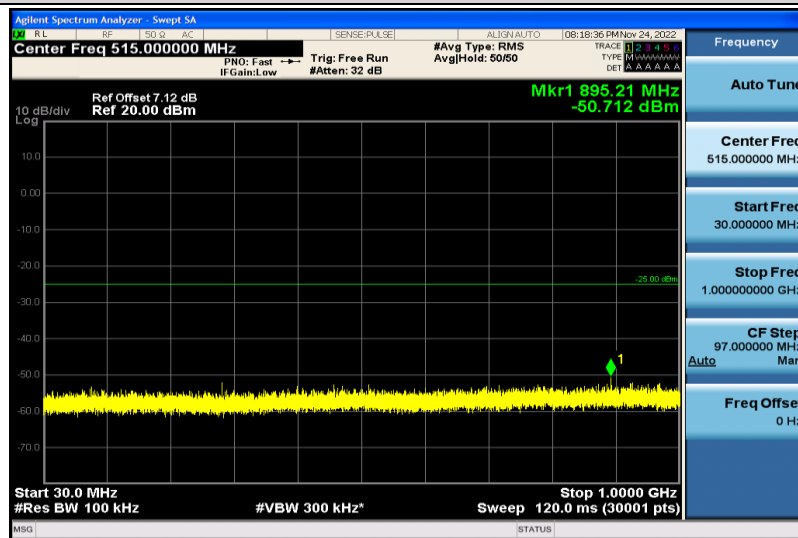
Band7-10MHz-QPSK-20800-1RB#0-30~1000MHz
