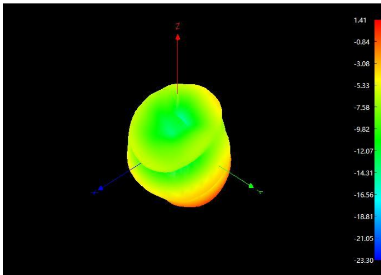
2450MHz 3D
