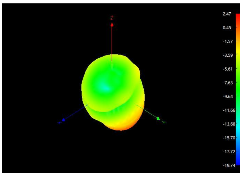
2500MHz 3D
