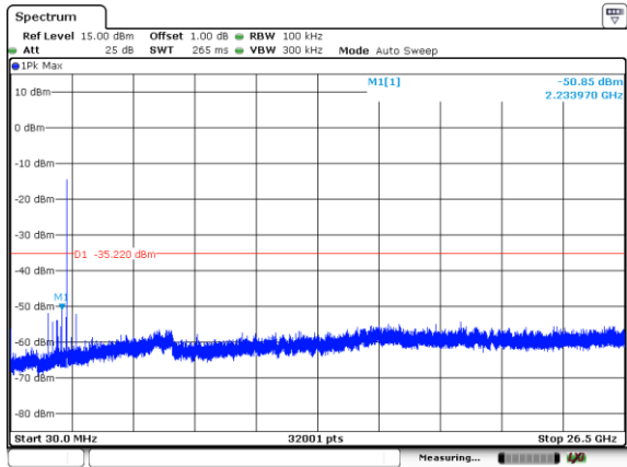
CH06-SE
