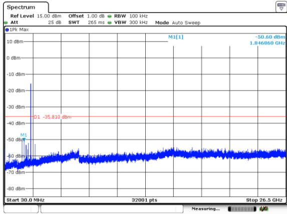
CH11-SE
