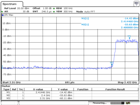
CH01-Bandedge
