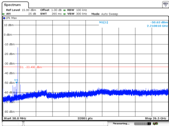
CH01-SE
