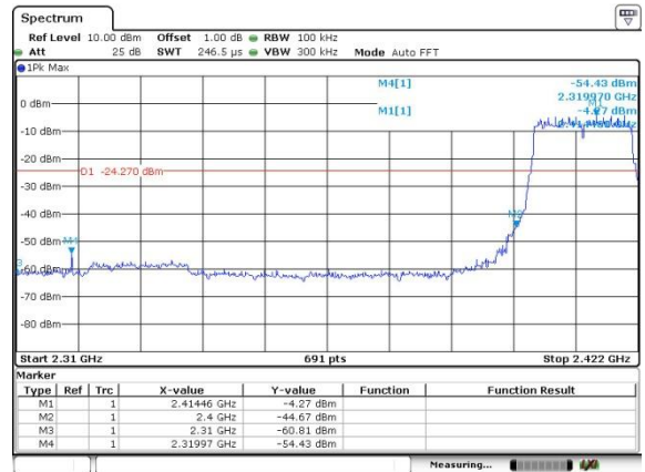
CH01-Bandedge
