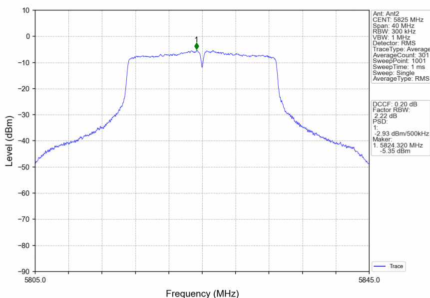
802.11n(HT20)_HCH_5825MHz_Ant2_NTNV
