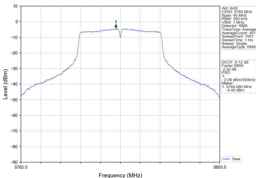
802.11a_MCH_5785MHz_Ant2_NTNV
