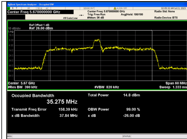
IEEE 802.11ax Channel 134 40MHz_Antenna 0_RU&Index 26RU8
