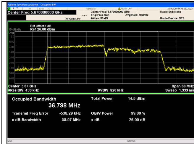
IEEE 802.11ax Channel 134 40MHz_Antenna 0 RU&Index 242RU61
