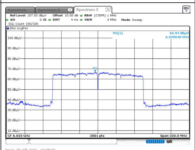
802.11be / 160MHz / 6025MHz / Ch15
