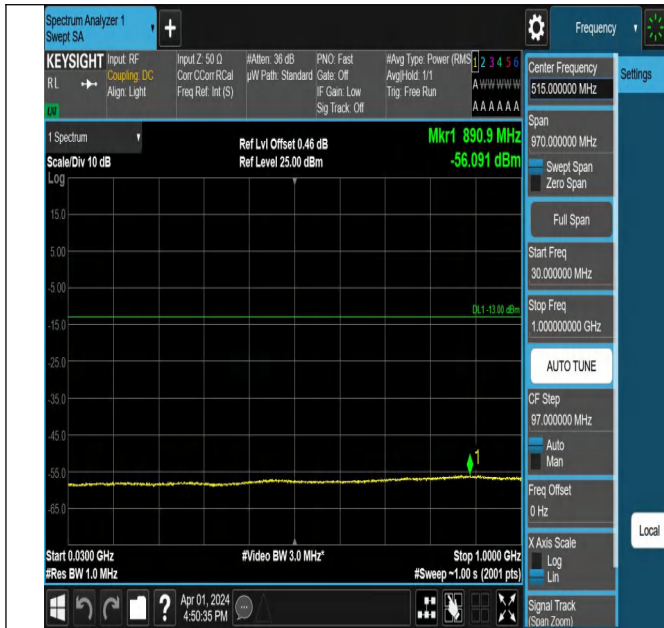
Band4-1312-1-30~1000MHz-PASS
