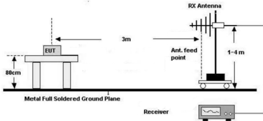
1GHz-18GHz(3m FAC)
