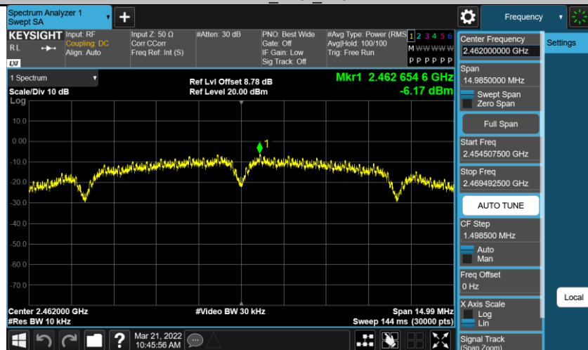
11B_Ant1_2462
