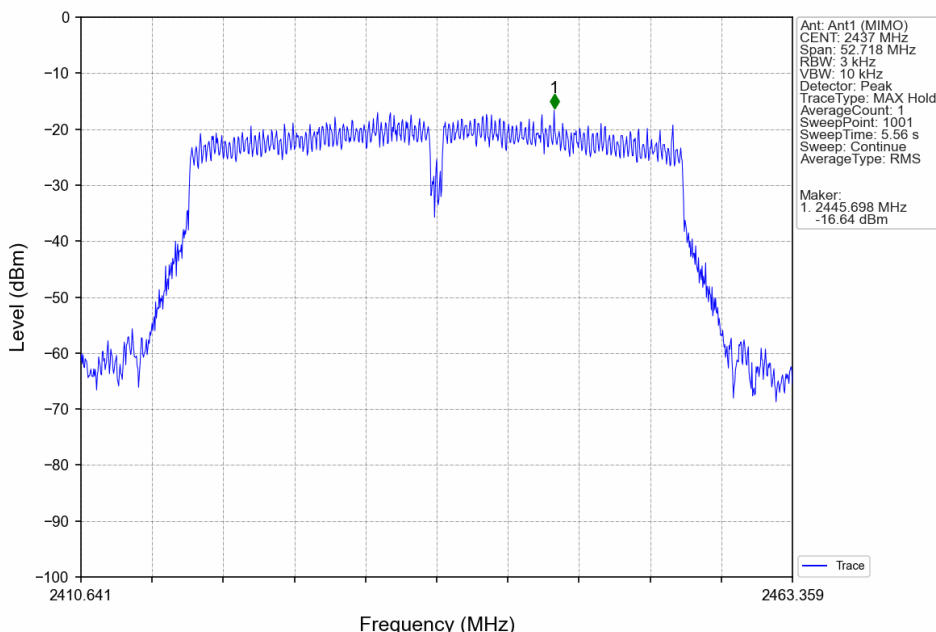
802.11n(HT40)_MCH_2437MHz_Ant1 (MIMO)_NTNV
